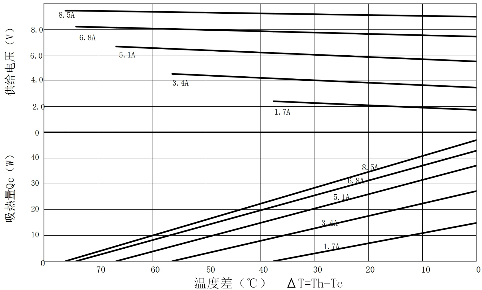
TEC1-B7108AC特性图 (Th=50°C)
