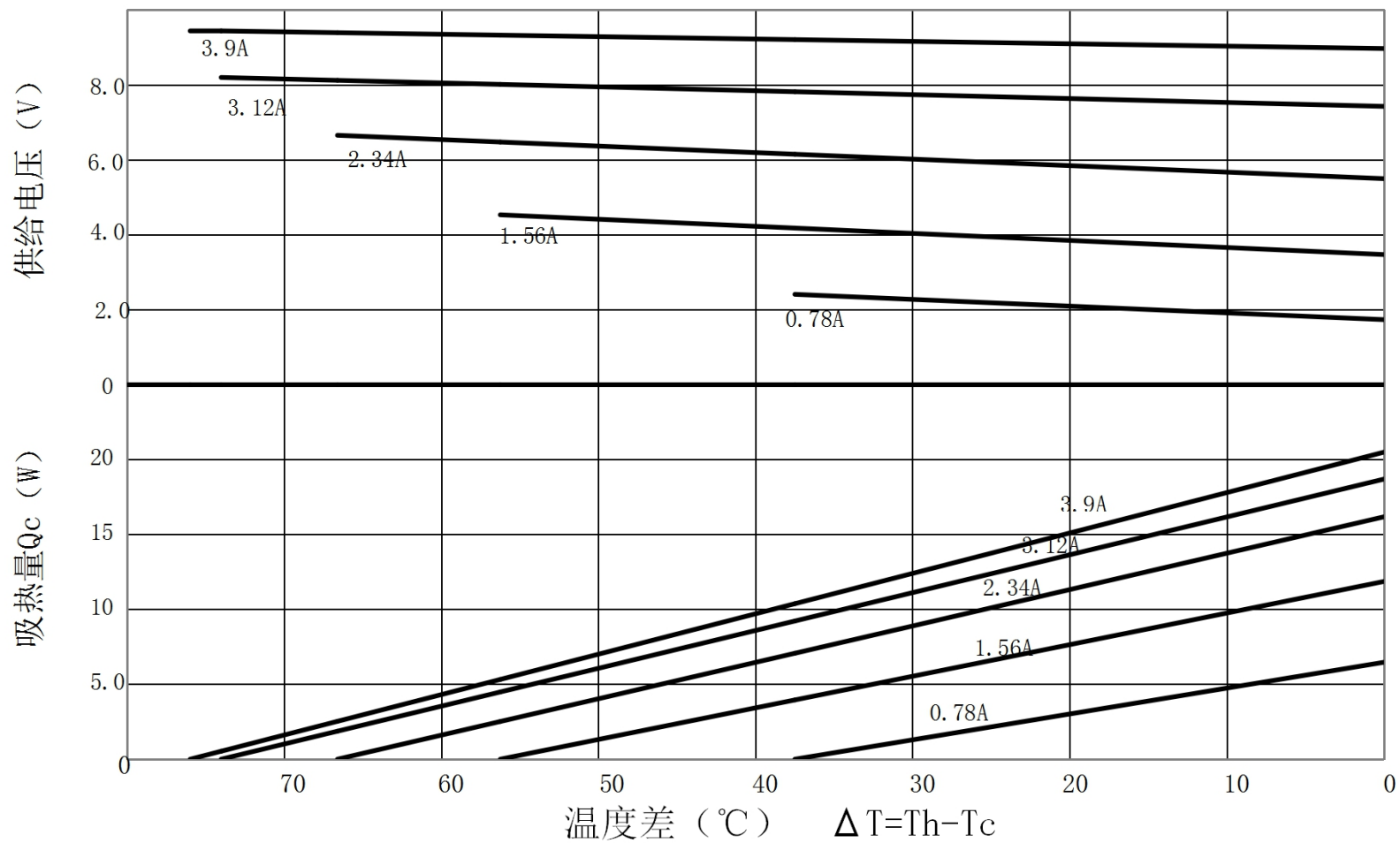
TEC1-B7104NC特性图 (Th=50°C)
