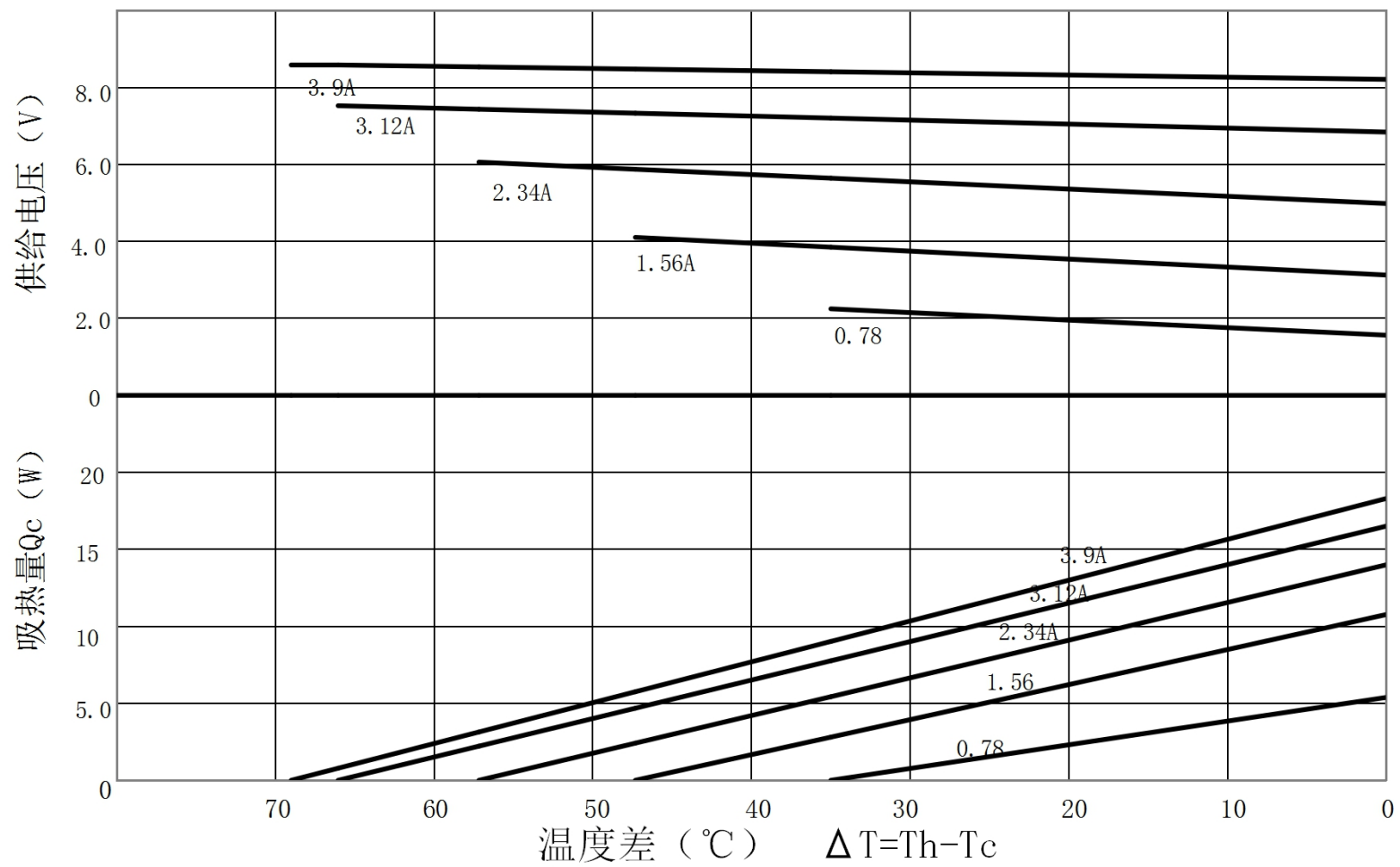
TEC1-B7104NC特性图 (Th=27°C)
