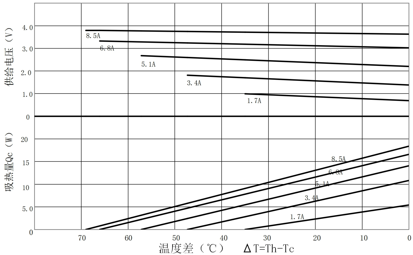
TEC1-B3108NC特性图 (Th=27°C)
