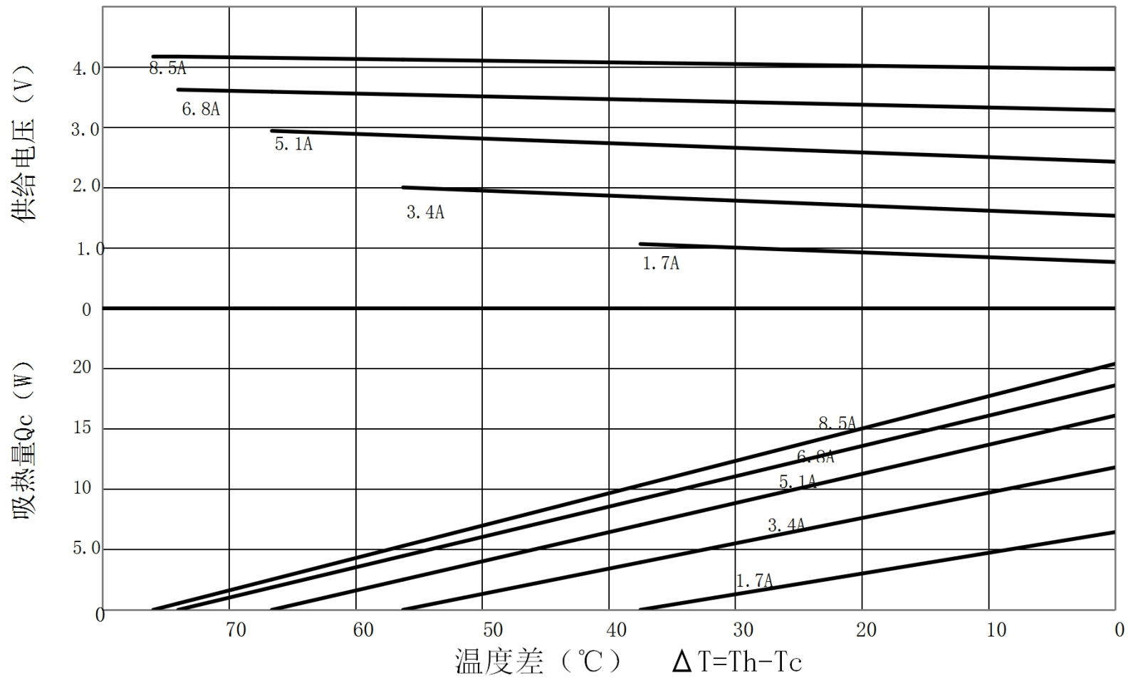
TEC1-B3108NC特性图 (Th=50°C)
