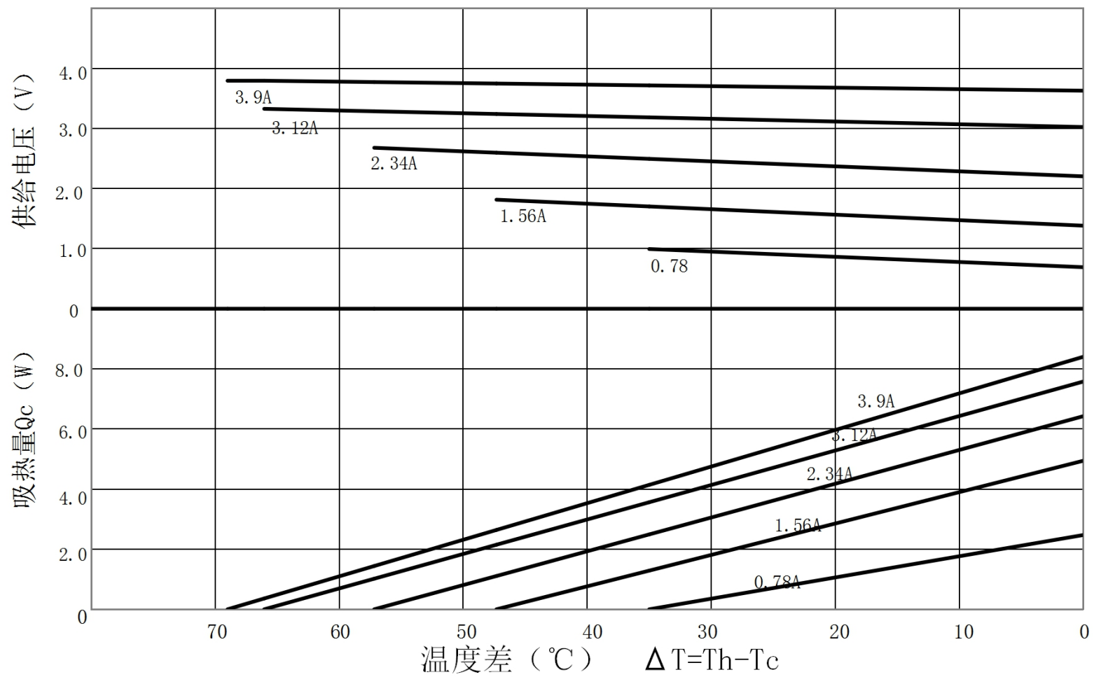
TEC1-B3104NC特性图 (Th=27°C)
