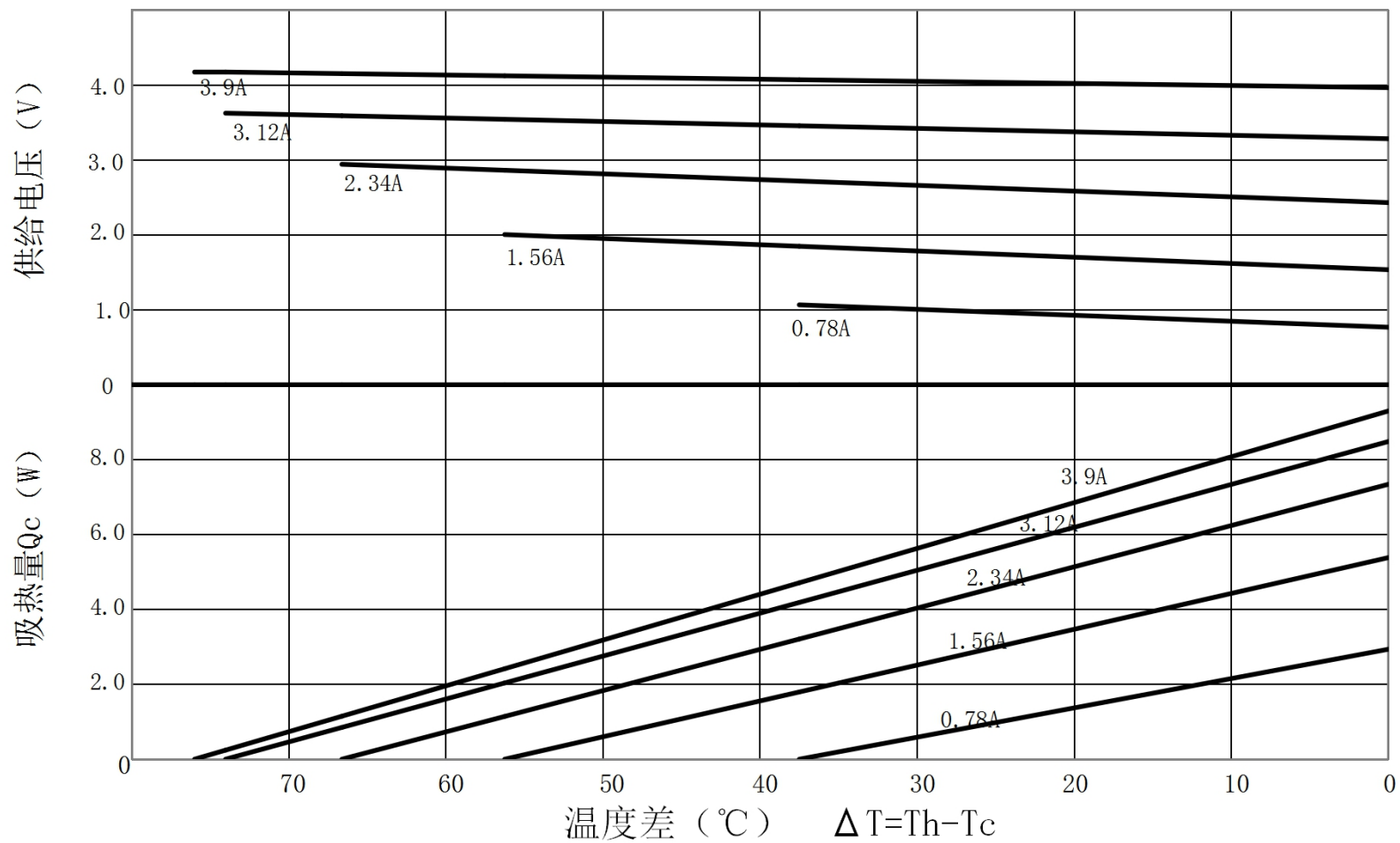
TEC1-B3104NC特性图 (Th=50°C)
