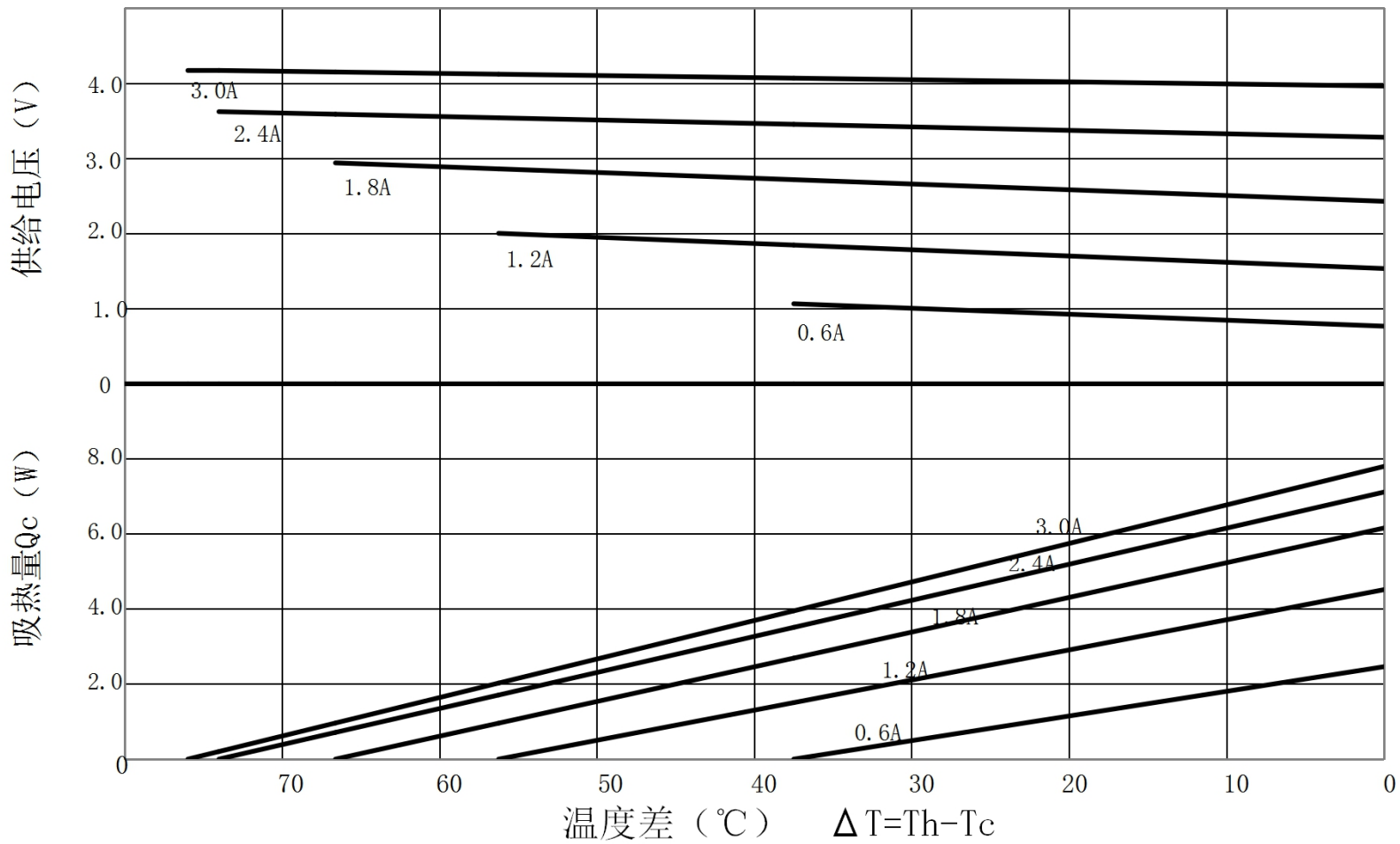
TEC1-B3103NC特性图 (Th=50°C)
