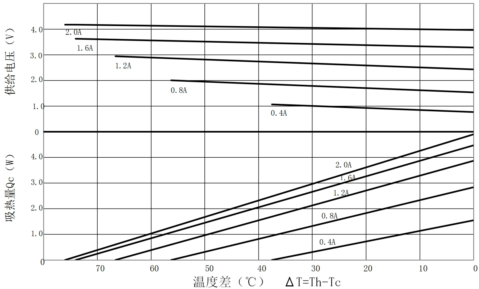
TEC1-B3102NC特性图 (Th=50°C)
