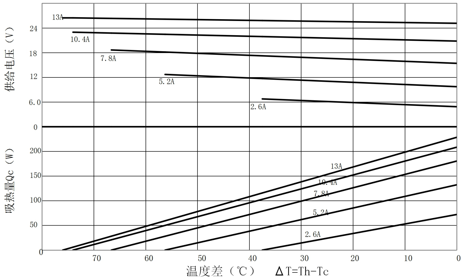
TEC1-B19913AC特性图 (Th=50°C)
