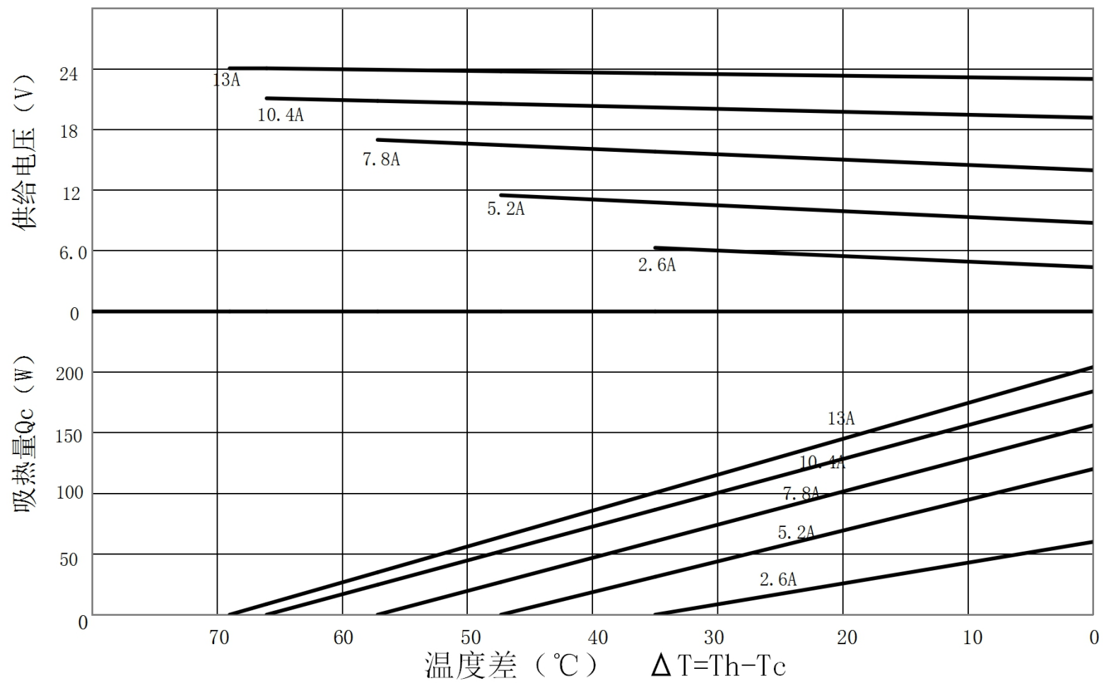
TEC1-B19913AC特性图 (Th=27°C)
