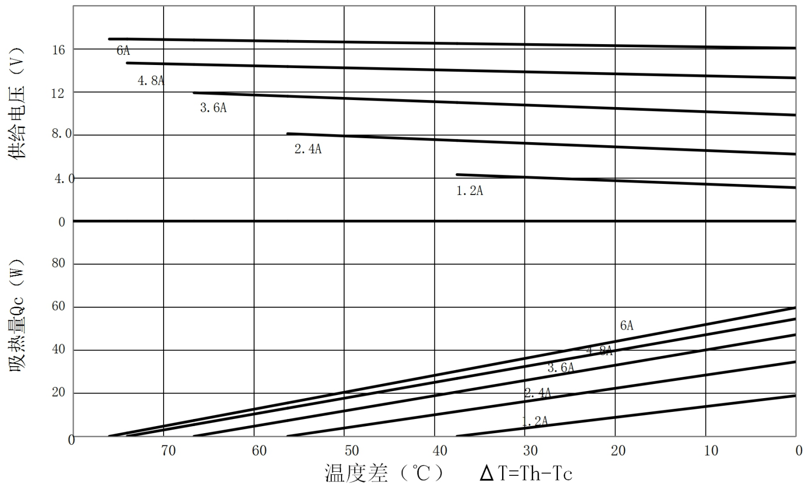
TEC1-B12707AC特性图 (Th=50°C)
