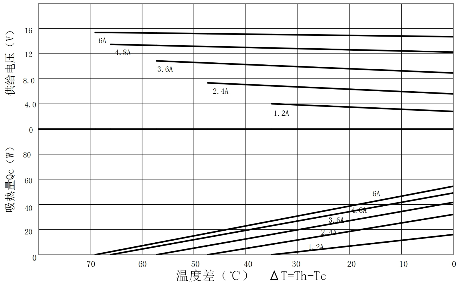
TEC1-B12707AC特性图 (Th=27°C)
