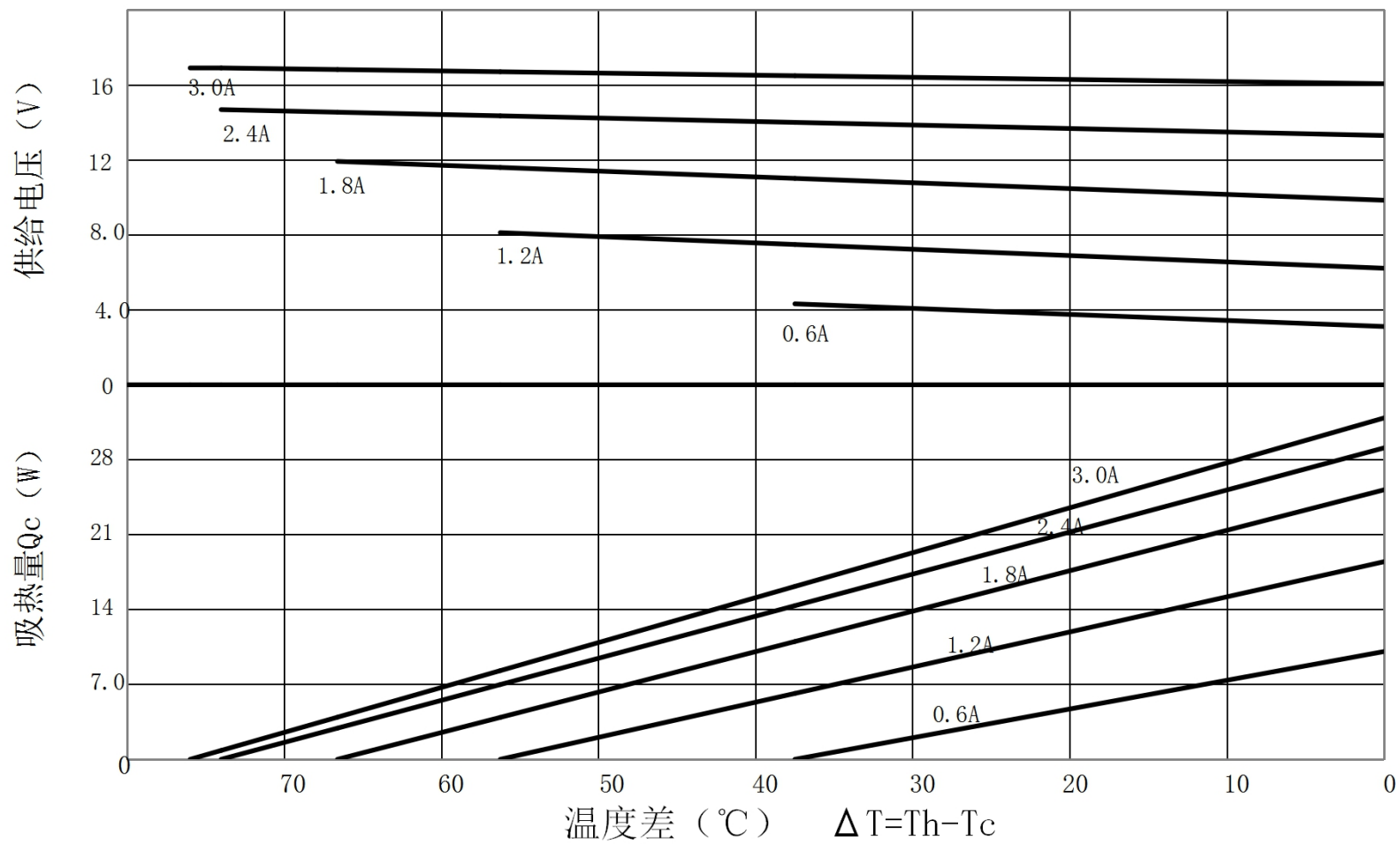
TEC1-B12703AC特性图 (Th=50°C)
