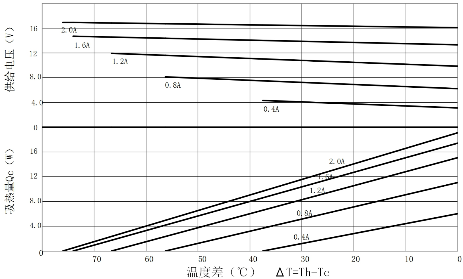
TEC1-B12702AC特性图 (Th=50°C)
