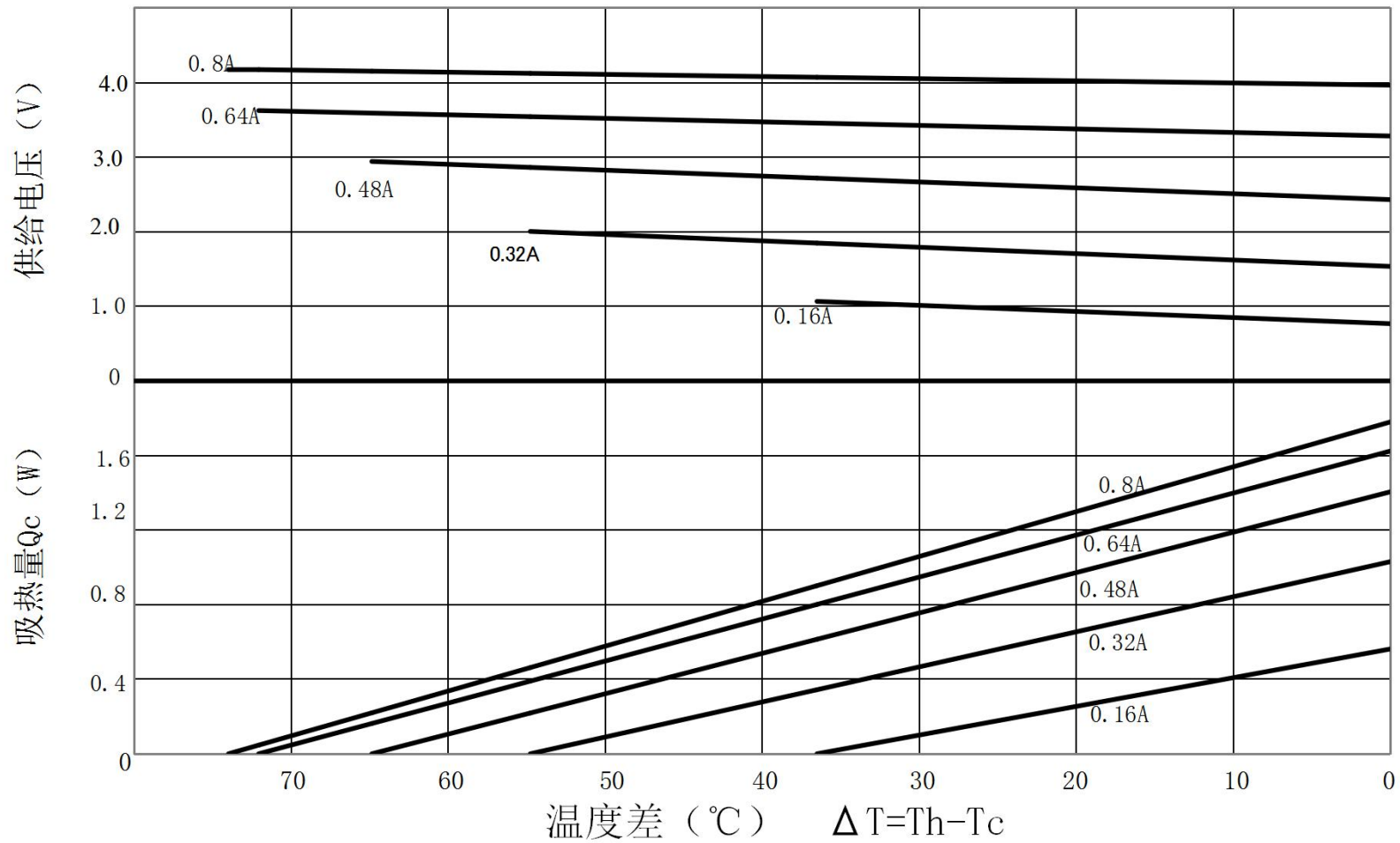
TEM1-B31008NC 特性图 (Th=50°C)
