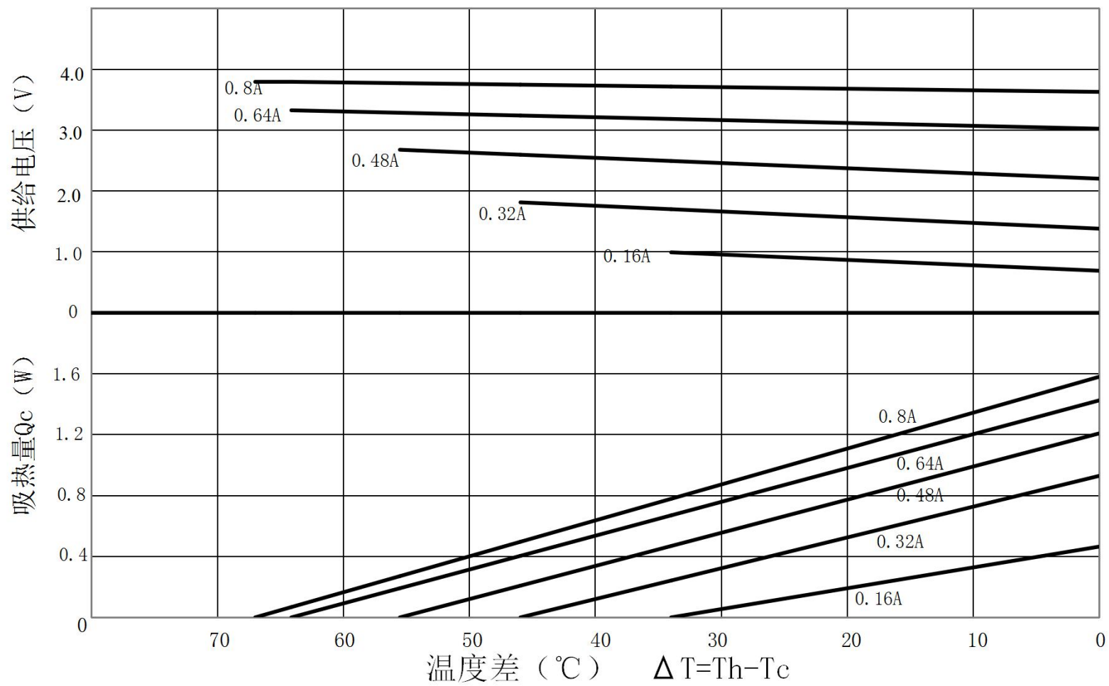
TEM1-B31008NC 特性图 (Th=27°C)
