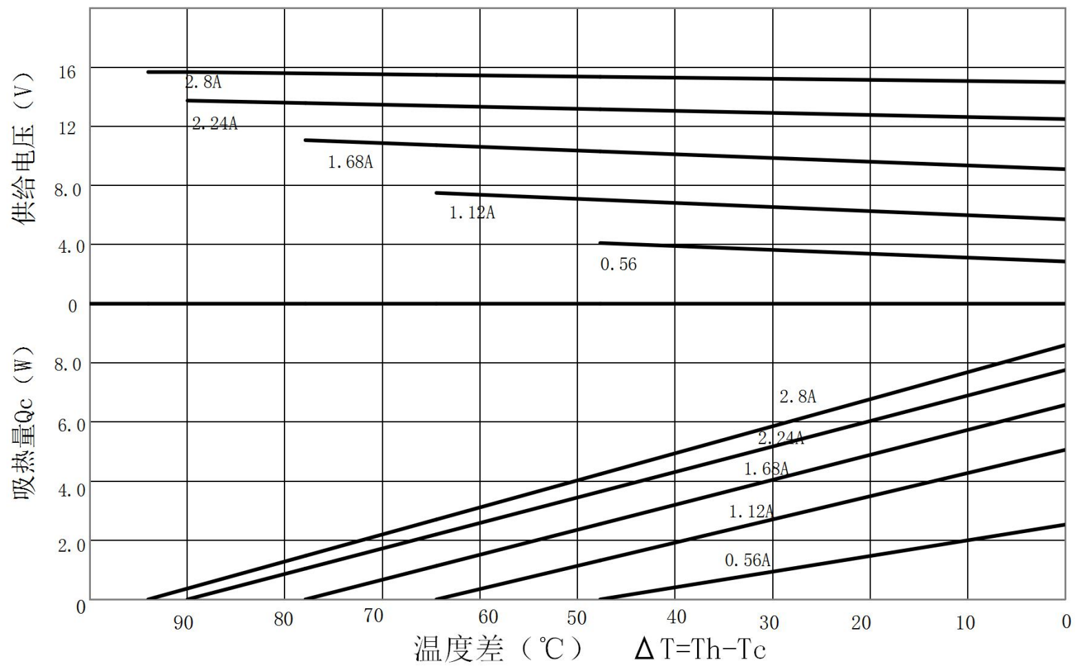
TEC2-B15828NC特性图 (Th=27°C)
