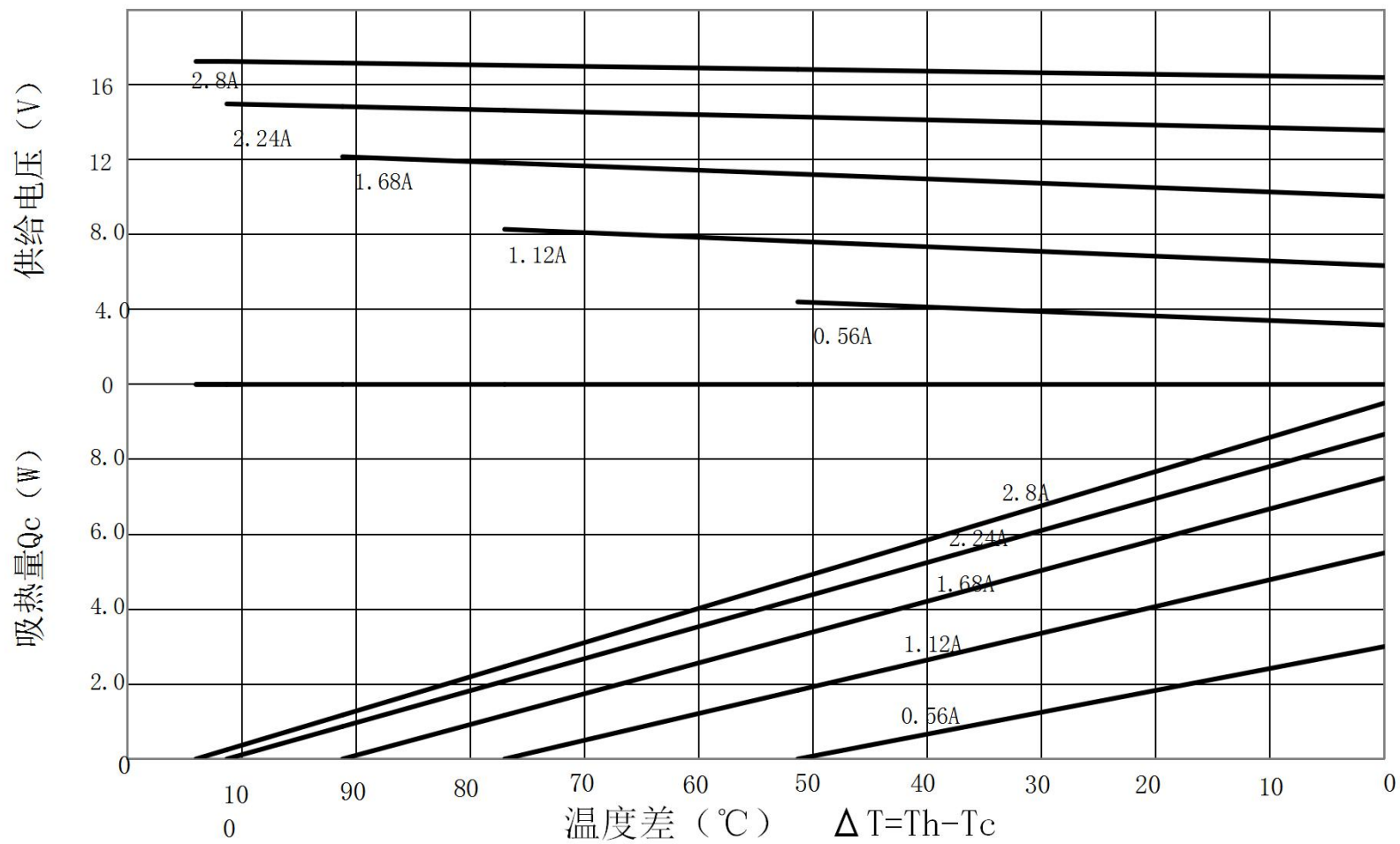
TEC2-B15828NC 特性图 (Th=50°C)
