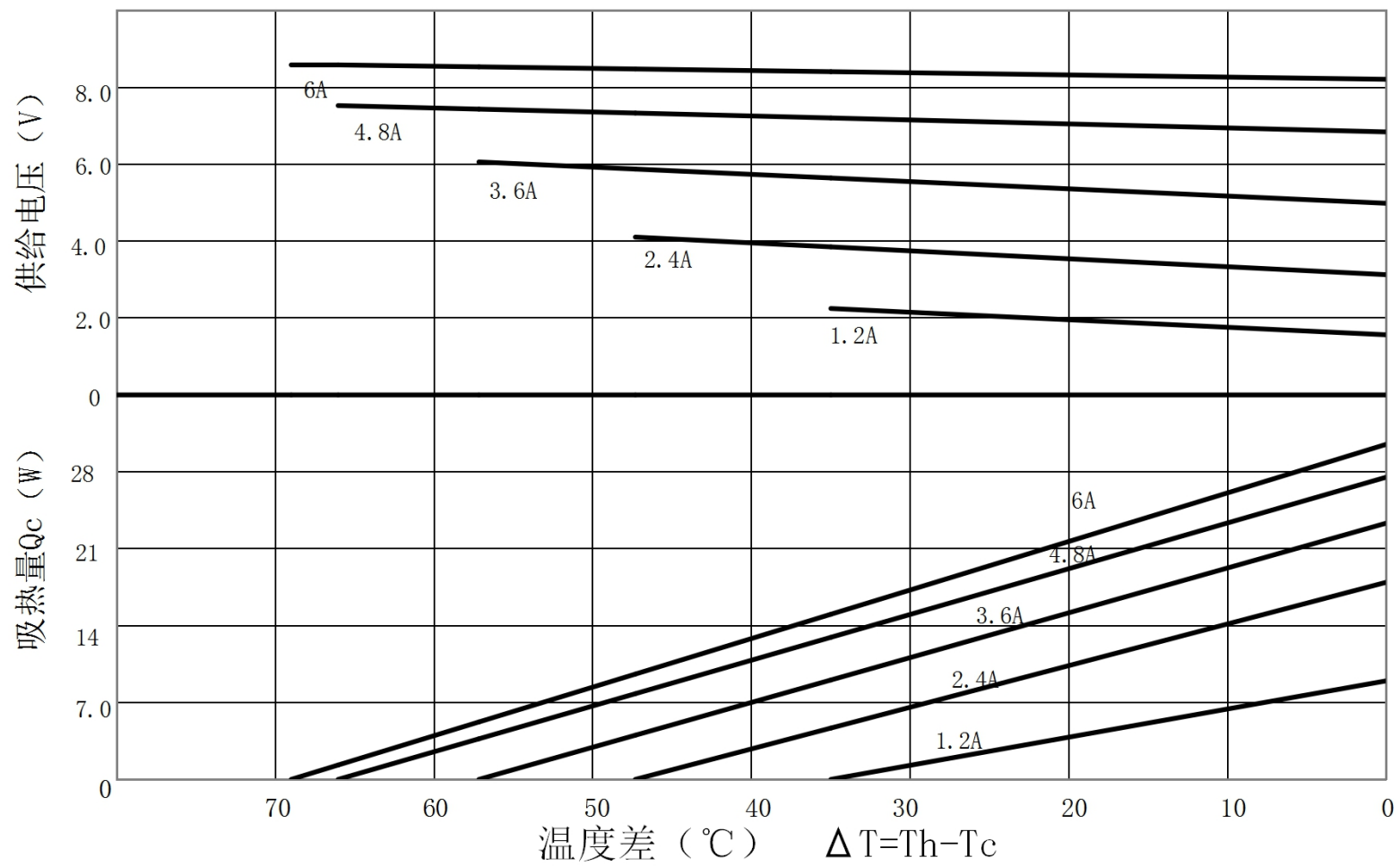
TEC1-B7107AC特性图 (Th=27°C)
