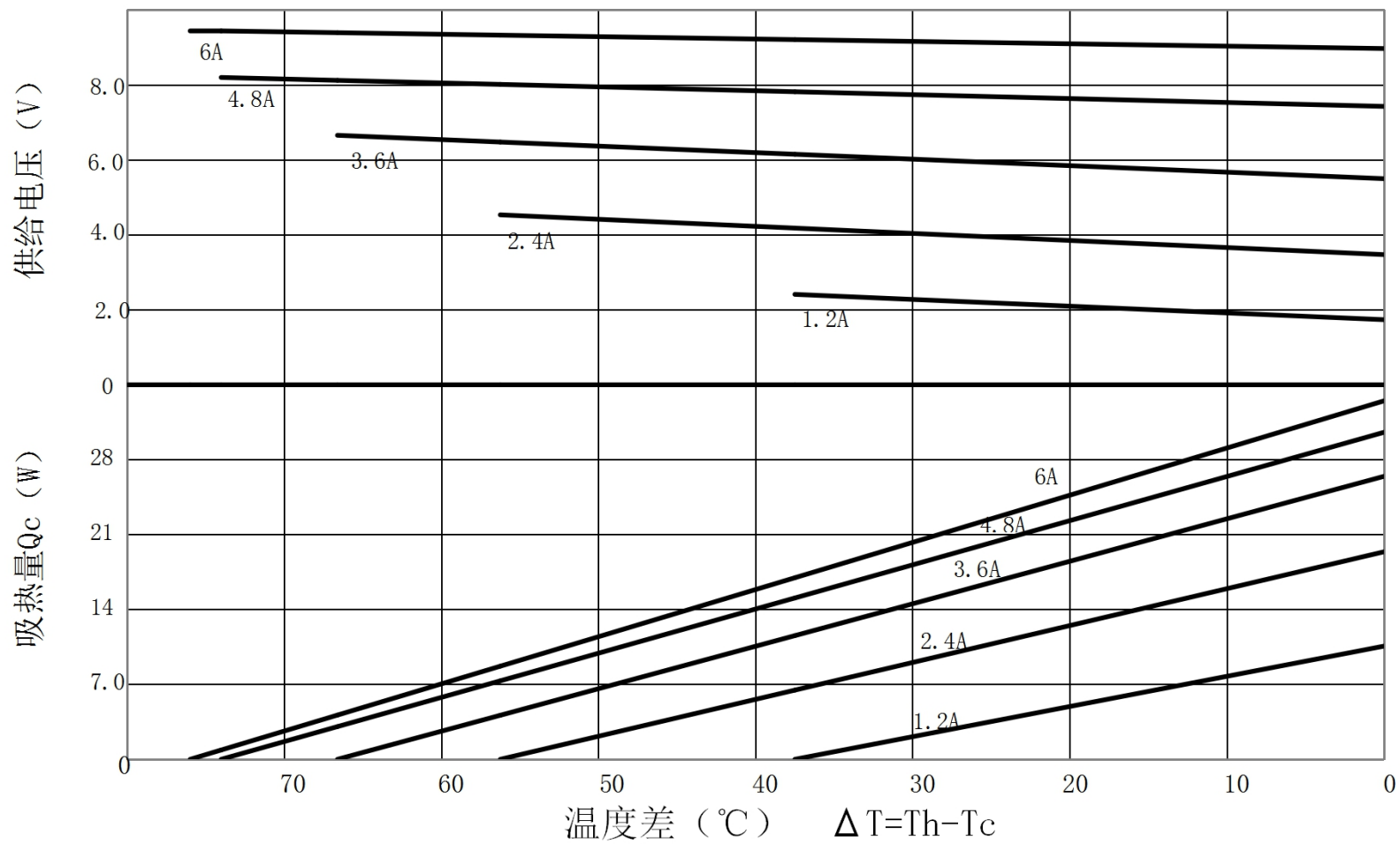
TEC1-B7107AC特性图 (Th=50°C)
