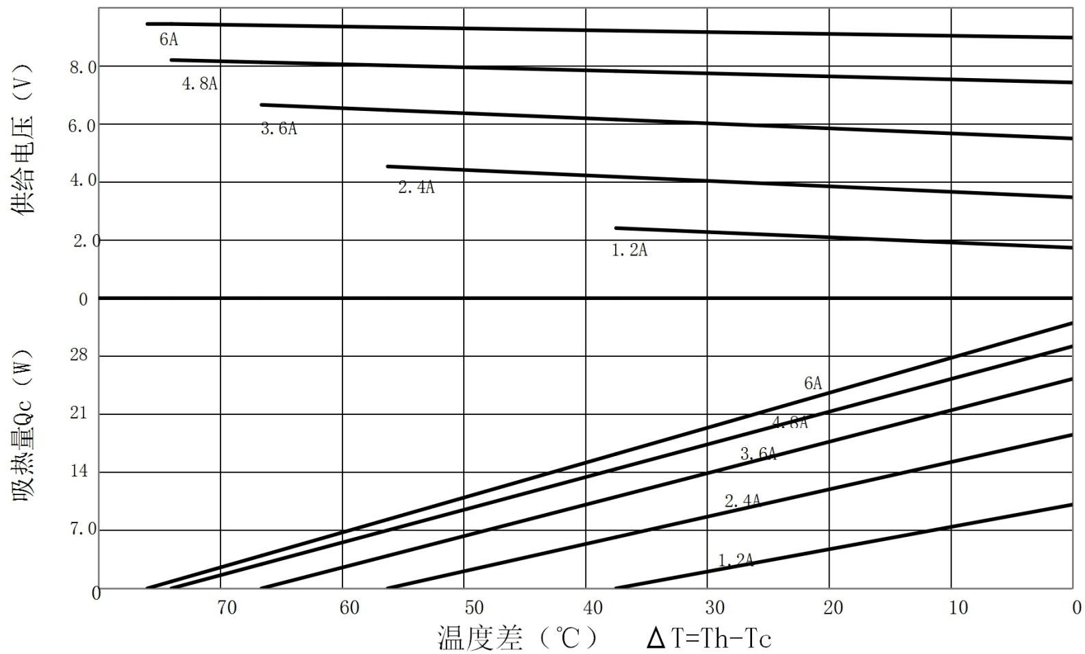
TEC1-B7106NC特性图 (Th=50°C)
