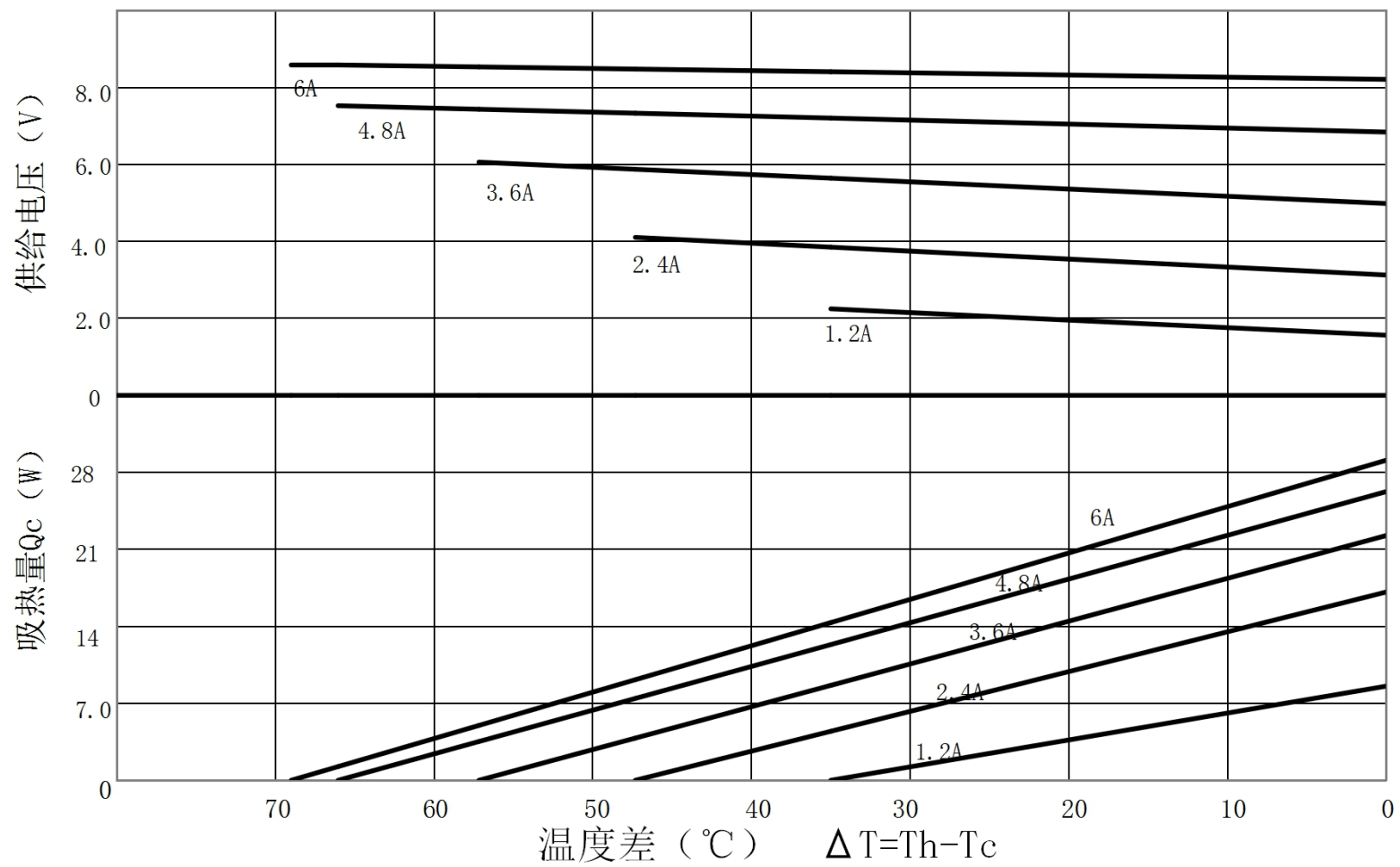
TEC1-B7106NC特性图 (Th=27°C)
