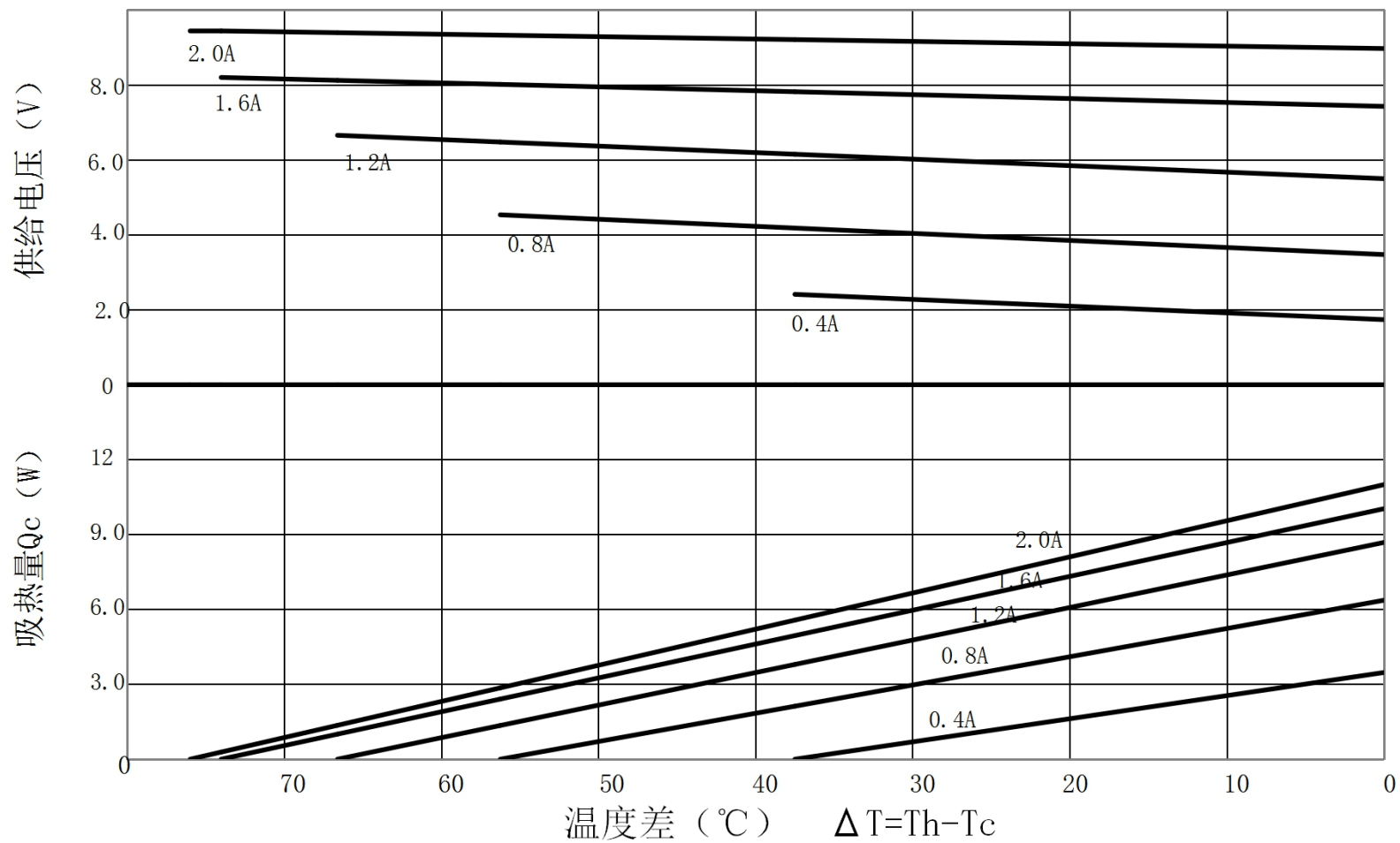
TEC1-B7102NC特性图 (Th=50°C)
