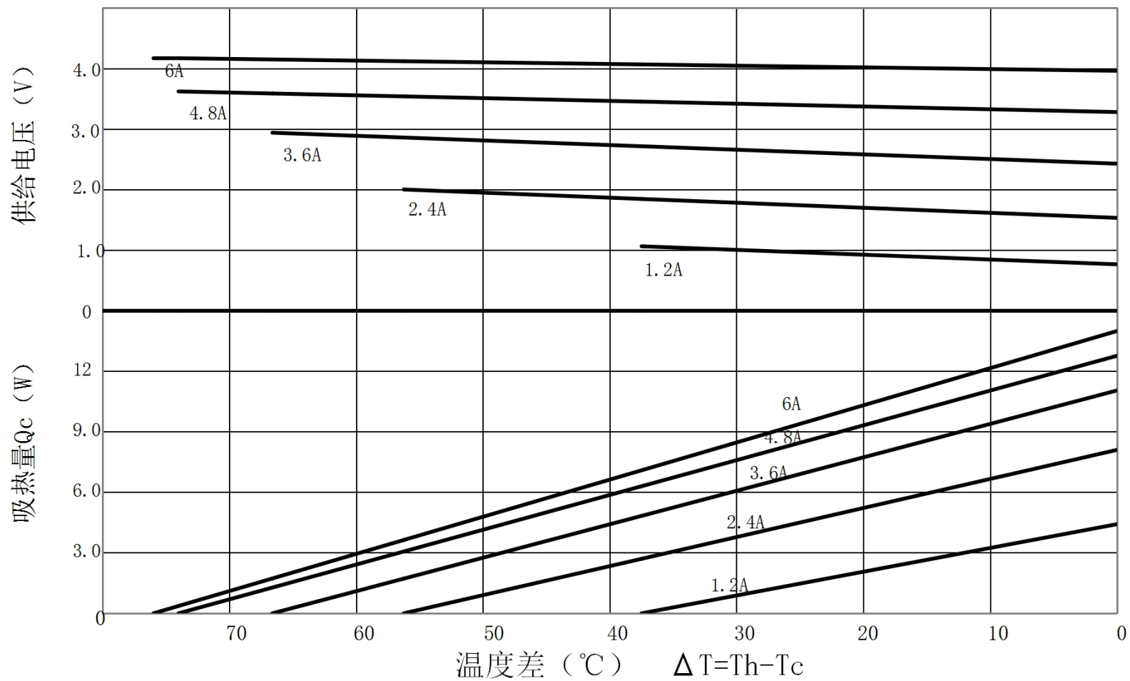
TEC1-B3106NC特性图 (Th=50°C)
