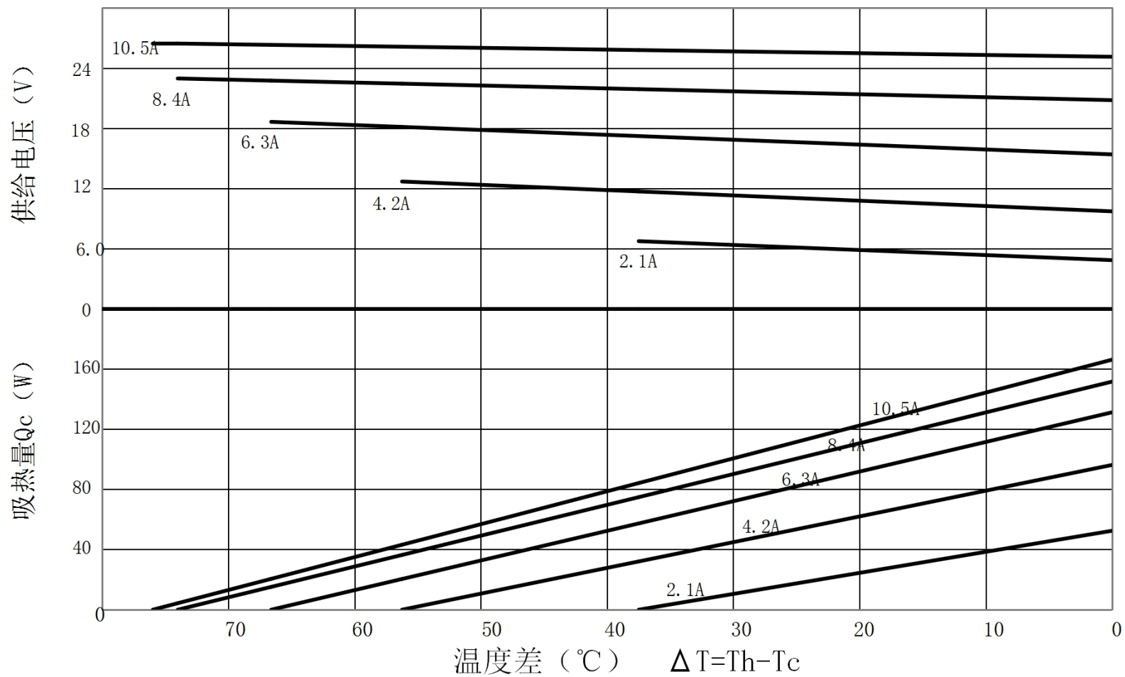
TEC1-B19910AC特性图 (Th=50°C)
