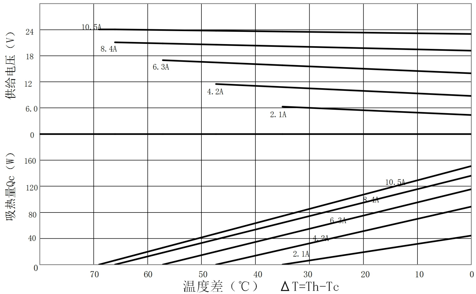
TEC1-B19910AC特性图 (Th=27°C)
