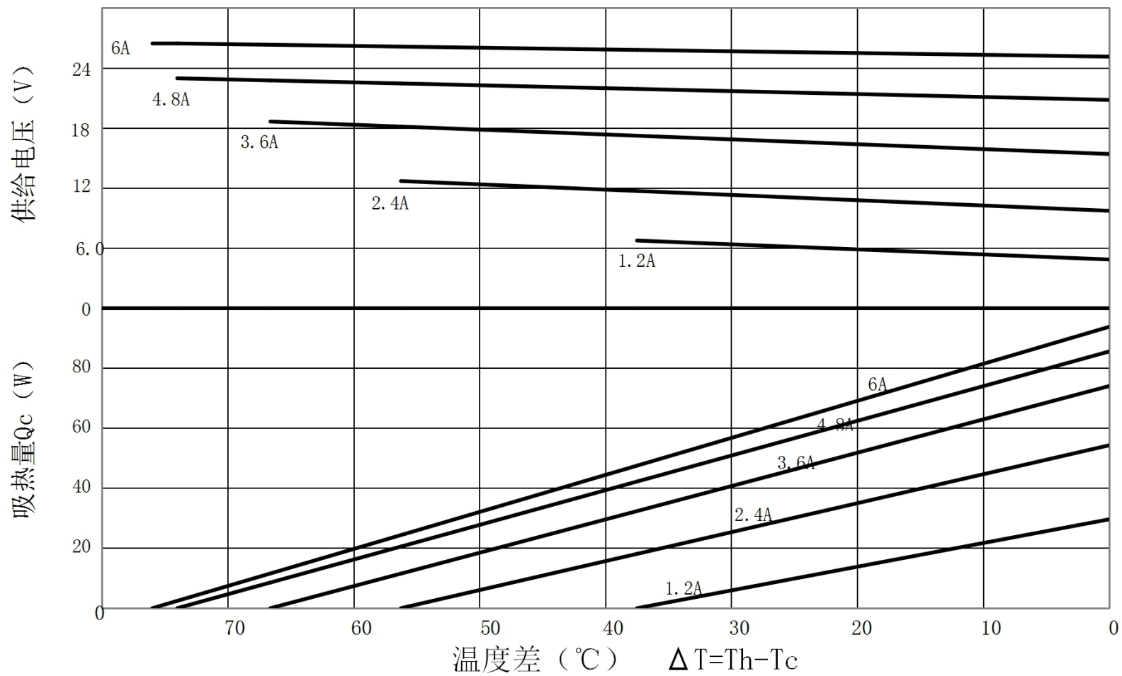
TEC1-B19906AC特性图 (Th=50°C)
