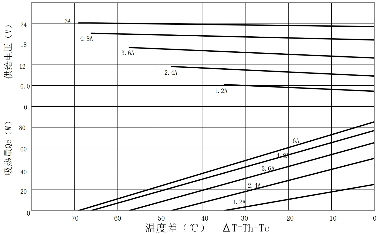
TEC1-B19906AC特性图 (Th=27°C)
