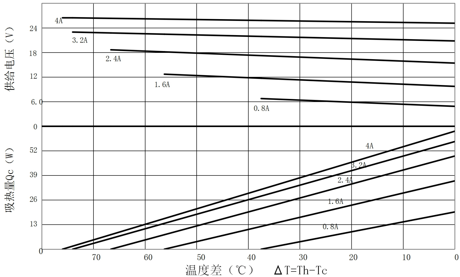
TEC1-B19904AC特性图 (Th=50°C)
