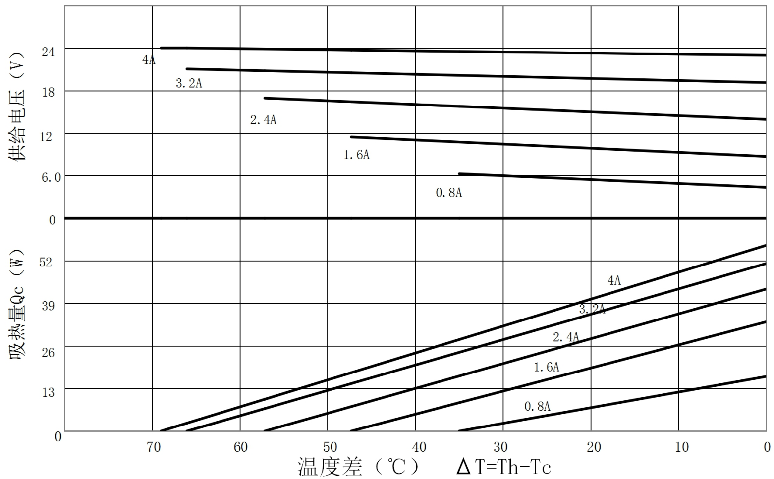
TEC1-B19904AC特性图 (Th=27°C)
