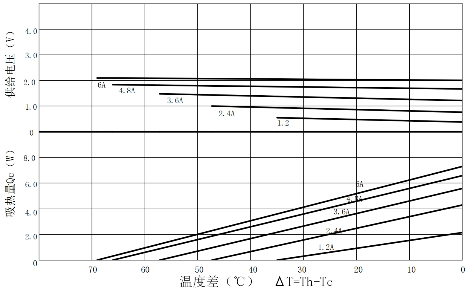
TEC1-B1707NC特性图 (Th=27°C)
