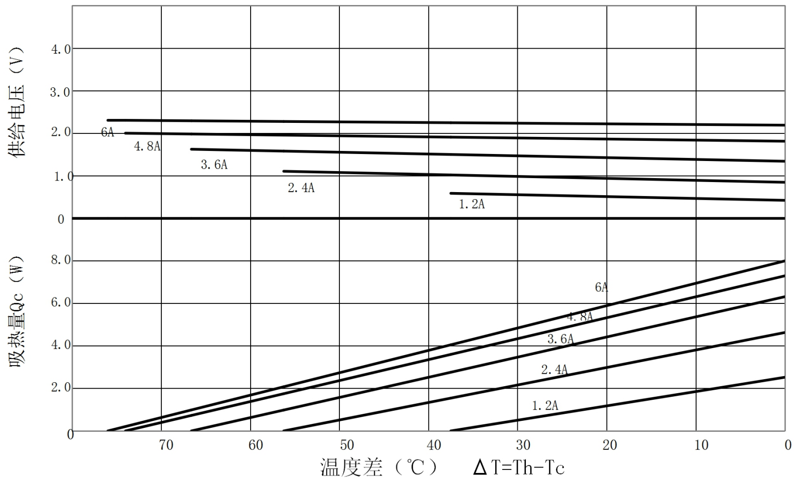
TEC1-B1707NC特性图 (Th=50°C)
