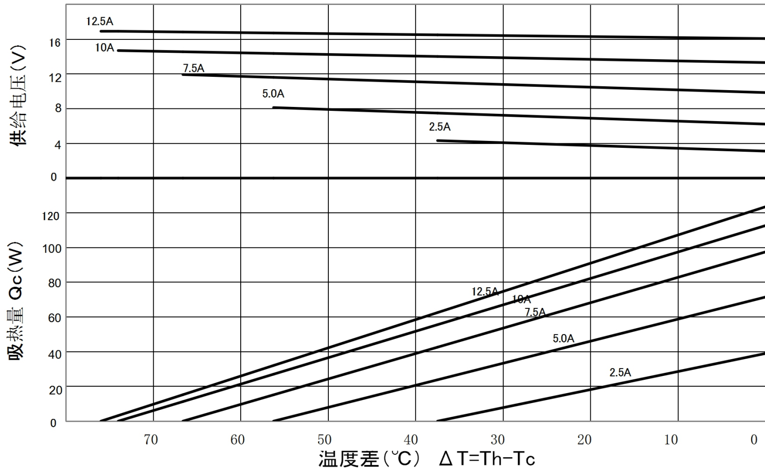
TEC1-B12712AC 特性图 (Th=50°C)
