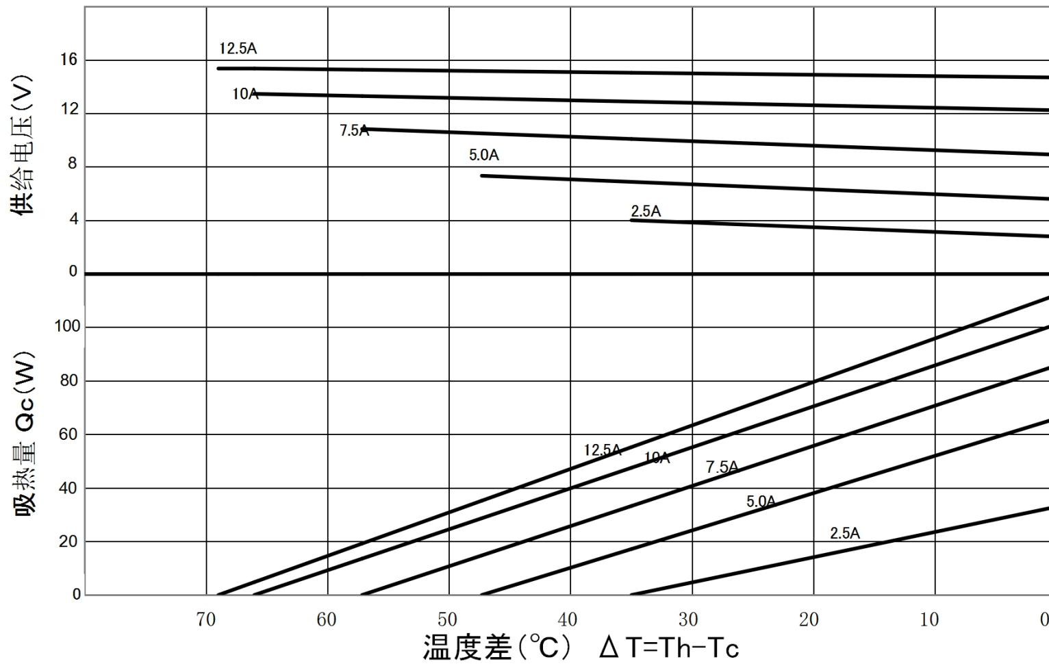
TEC1-B12712AC 特性图 (Th=27°C)
