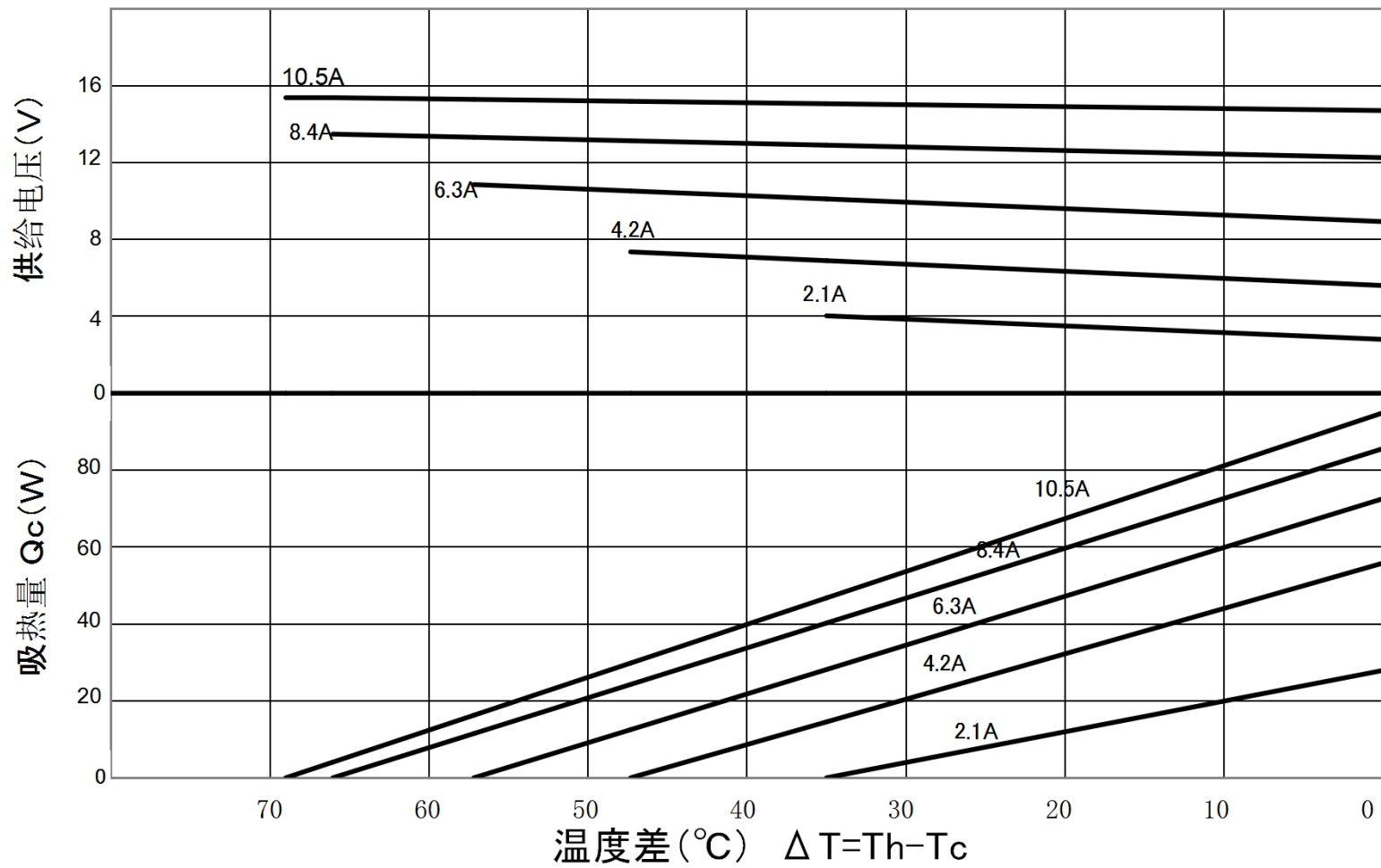
TEC1-B12710AC 特性图 (Th=27°C)
