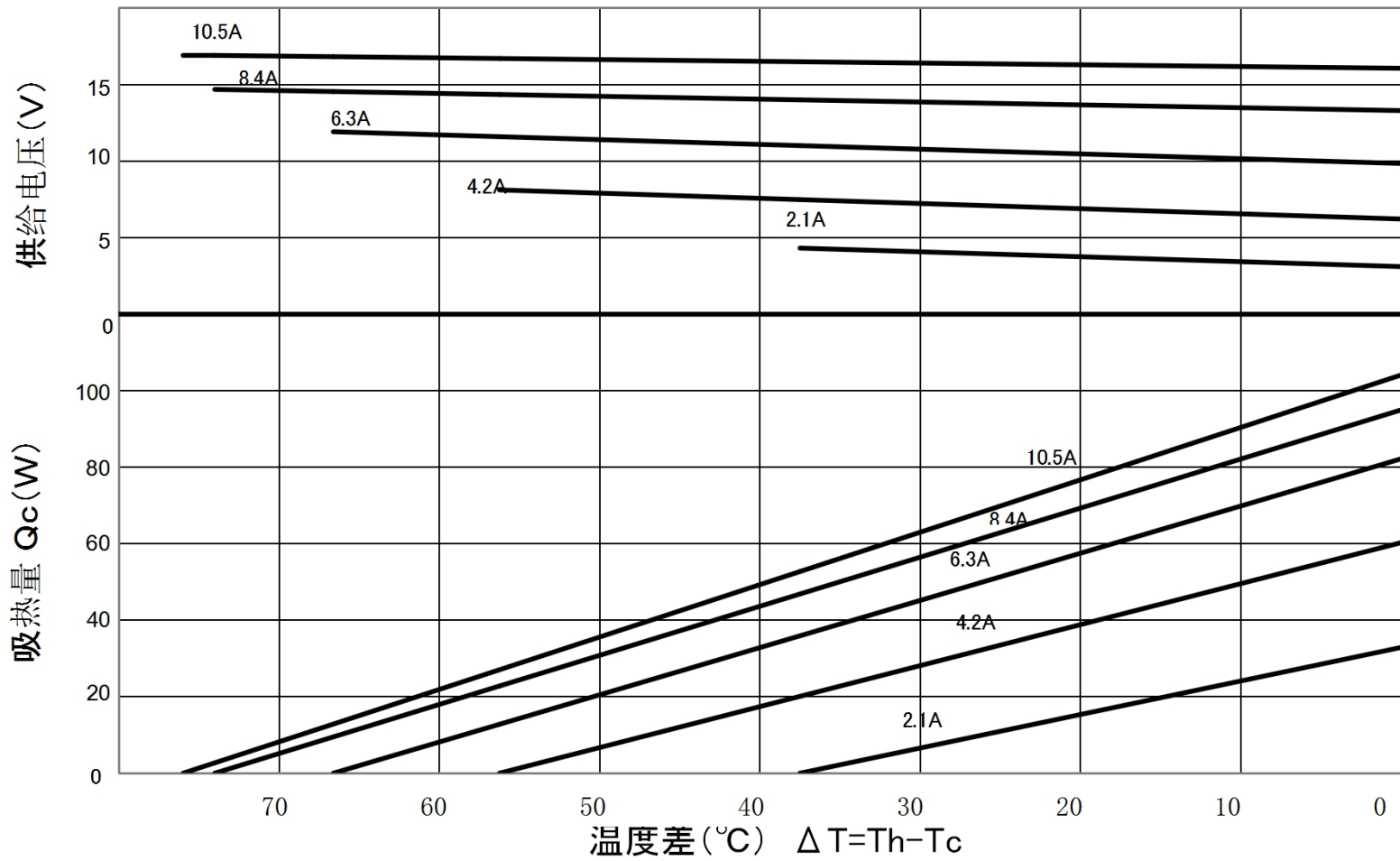
TEC1-B12710AC 特性图 (Th=50°C)
