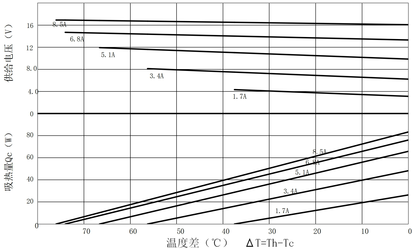
TEC1-B12708AC特性图 (Th=50°C)
