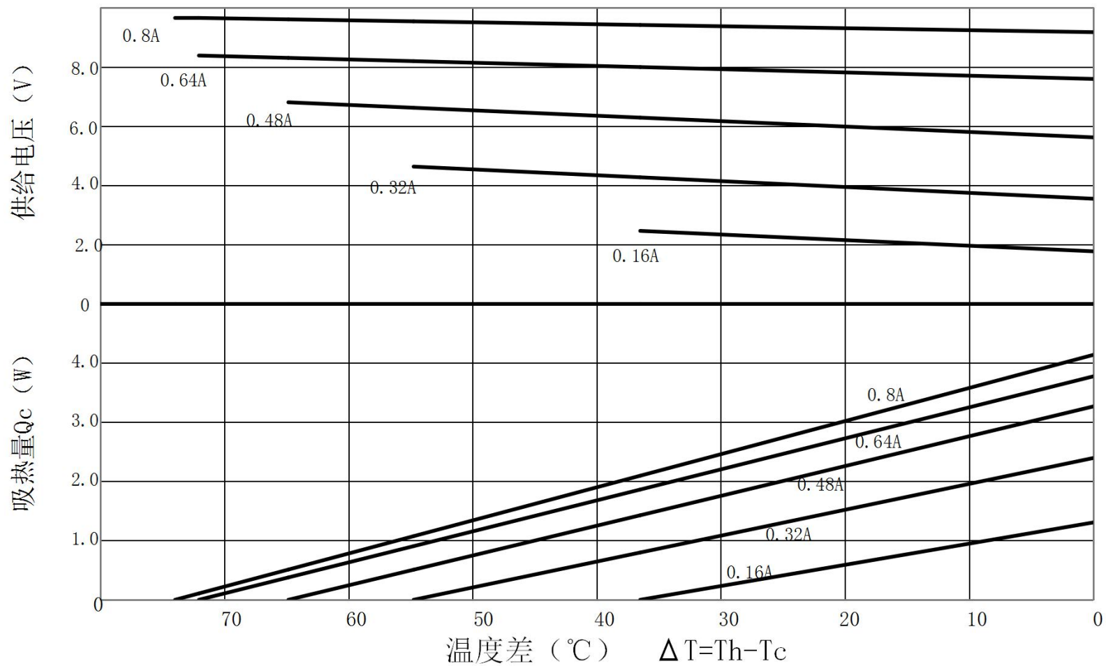
TEM1-B71008NC特性图 (Th=50°C)
