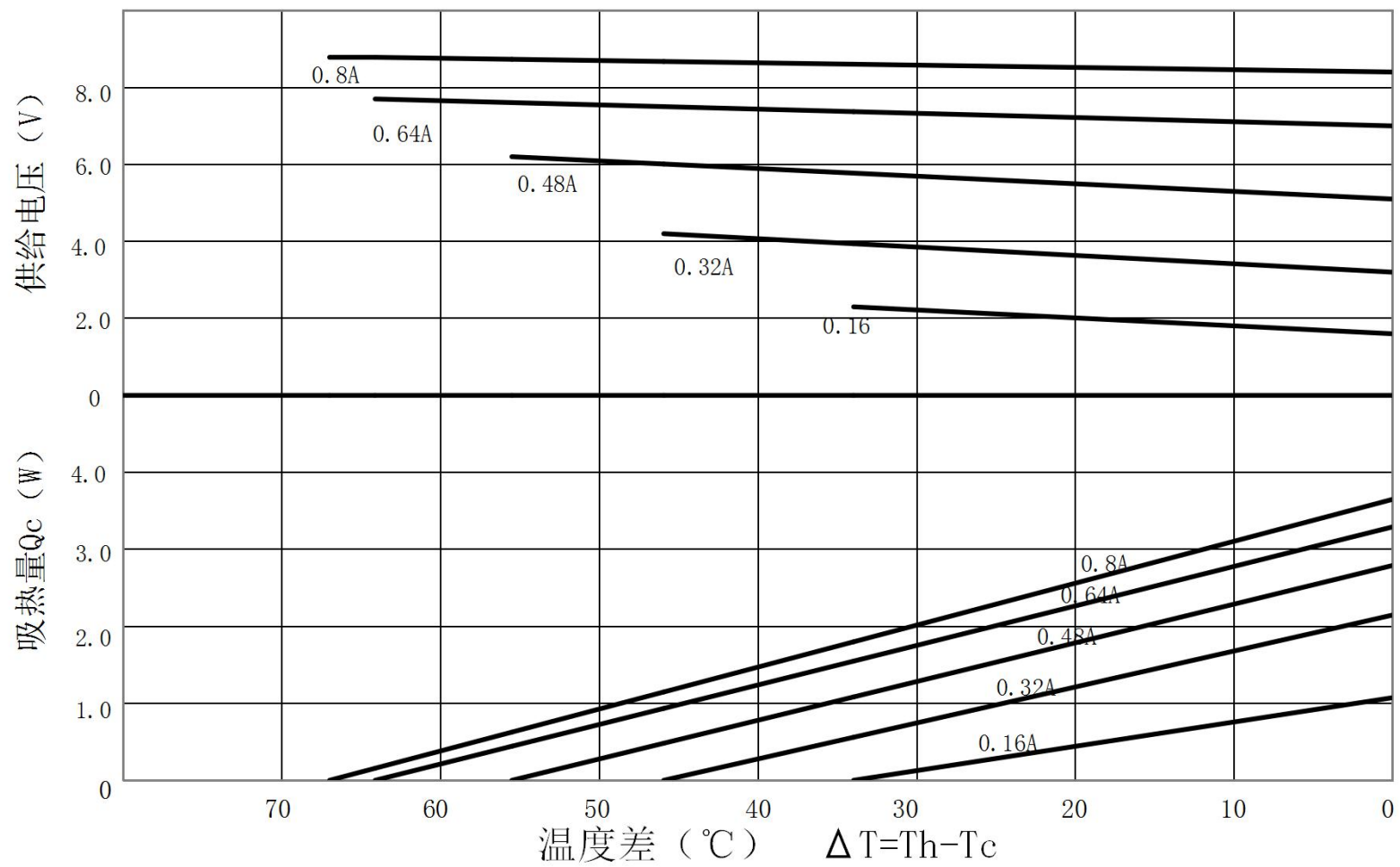
TEM1-B71008NC特性图 (Th=27°C)
