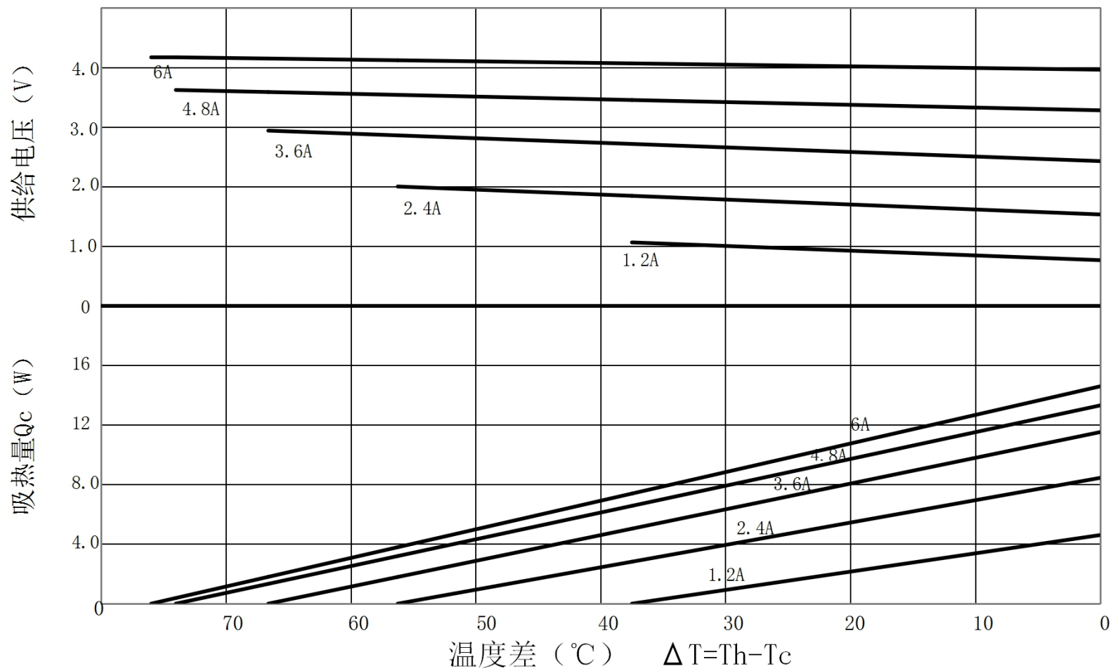
TEC1-3107NC特性图 (Th=50°C)
