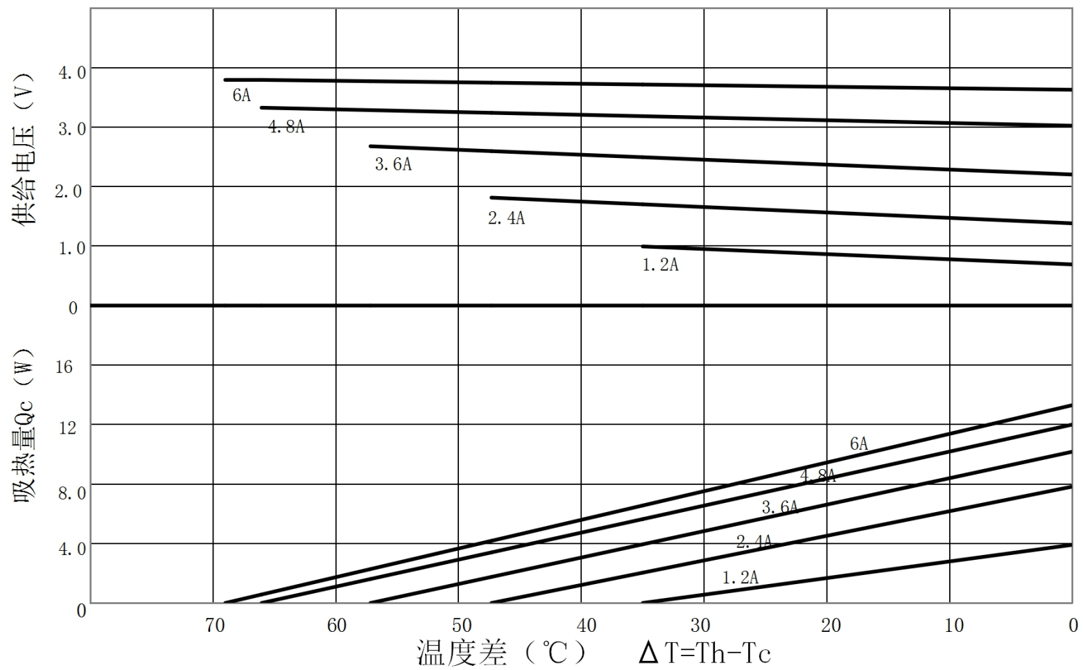
TEC1-B3107NC特性图 (Th=27°C)
