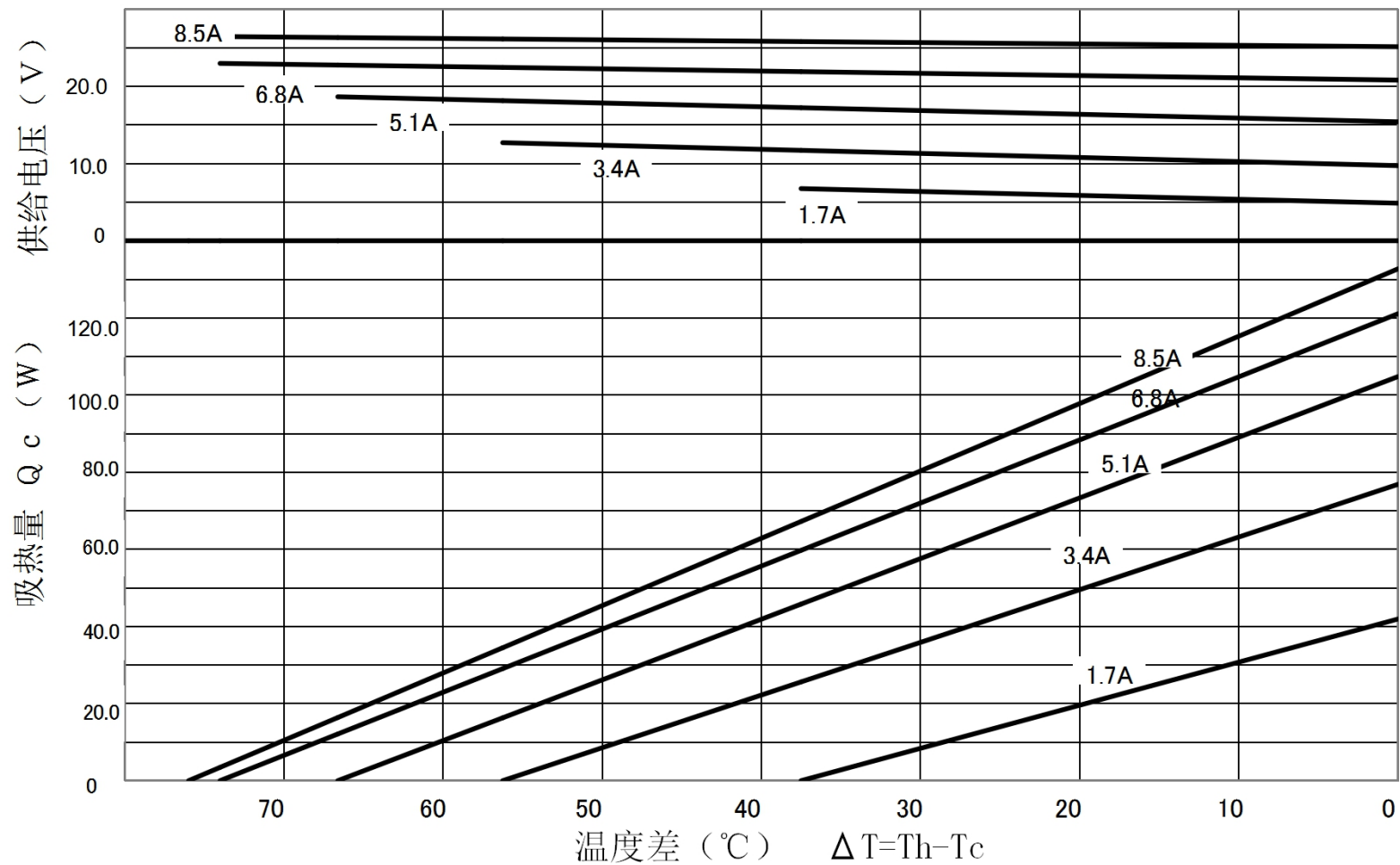
TEC1-B19908AC特性图 (Th=50°C)
