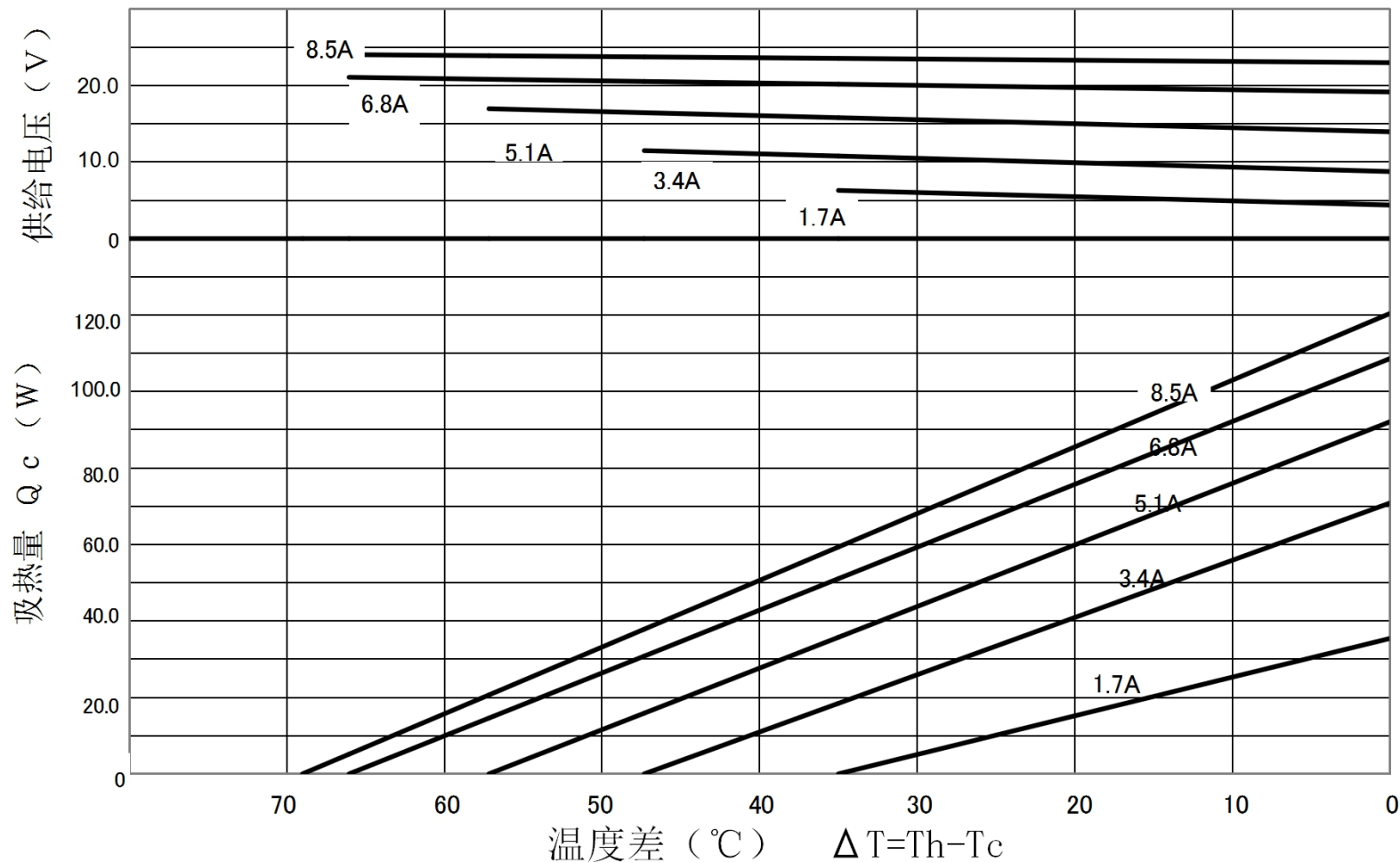
TEC1-B19908AC特性图 (Th=27°C)
