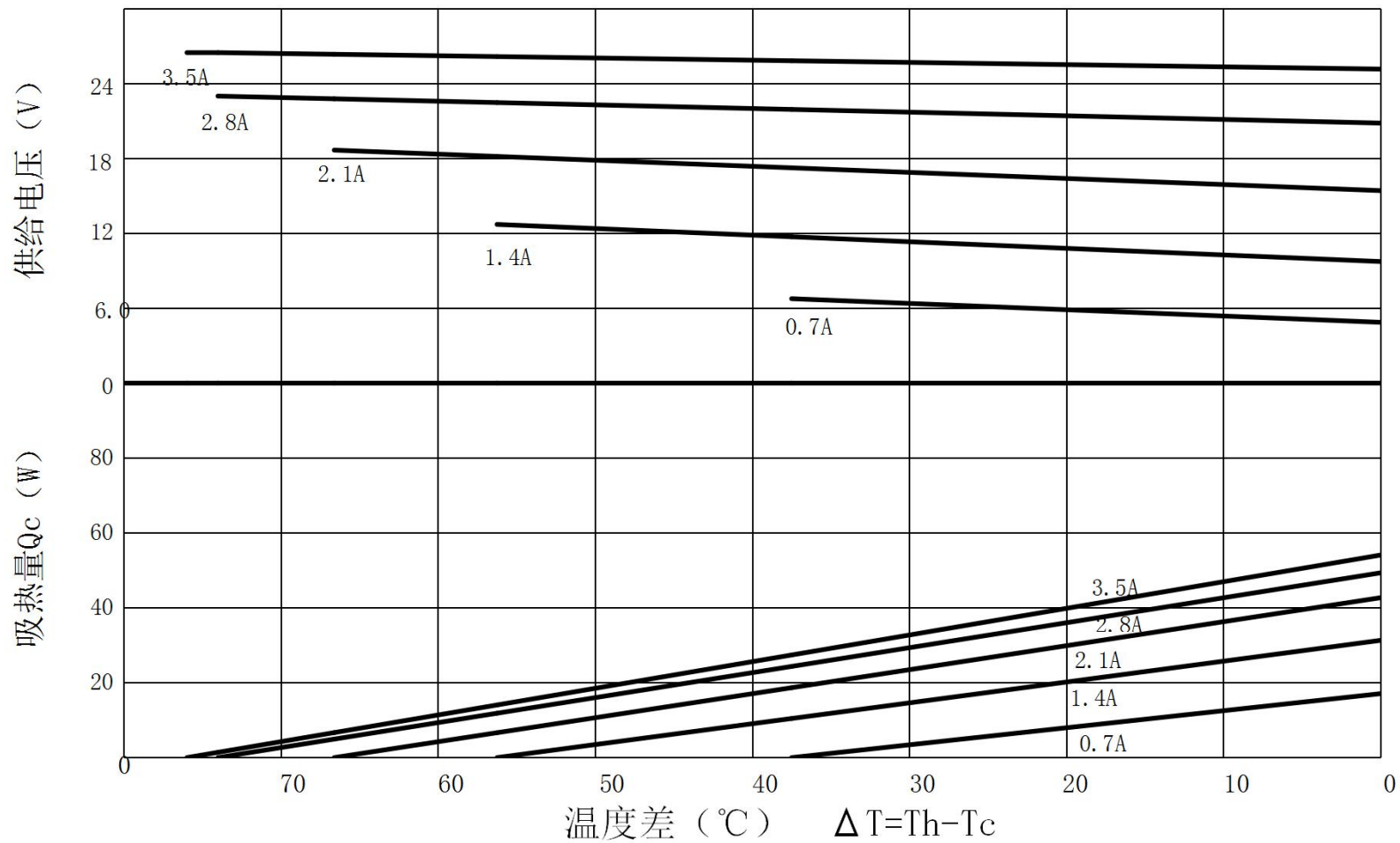
TEC1-B19903AC 特性图 (Th=50°C)
