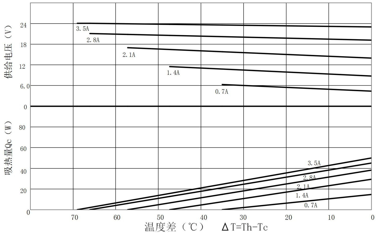
TEC1-B19903AC 特性图 (Th=27°C)
