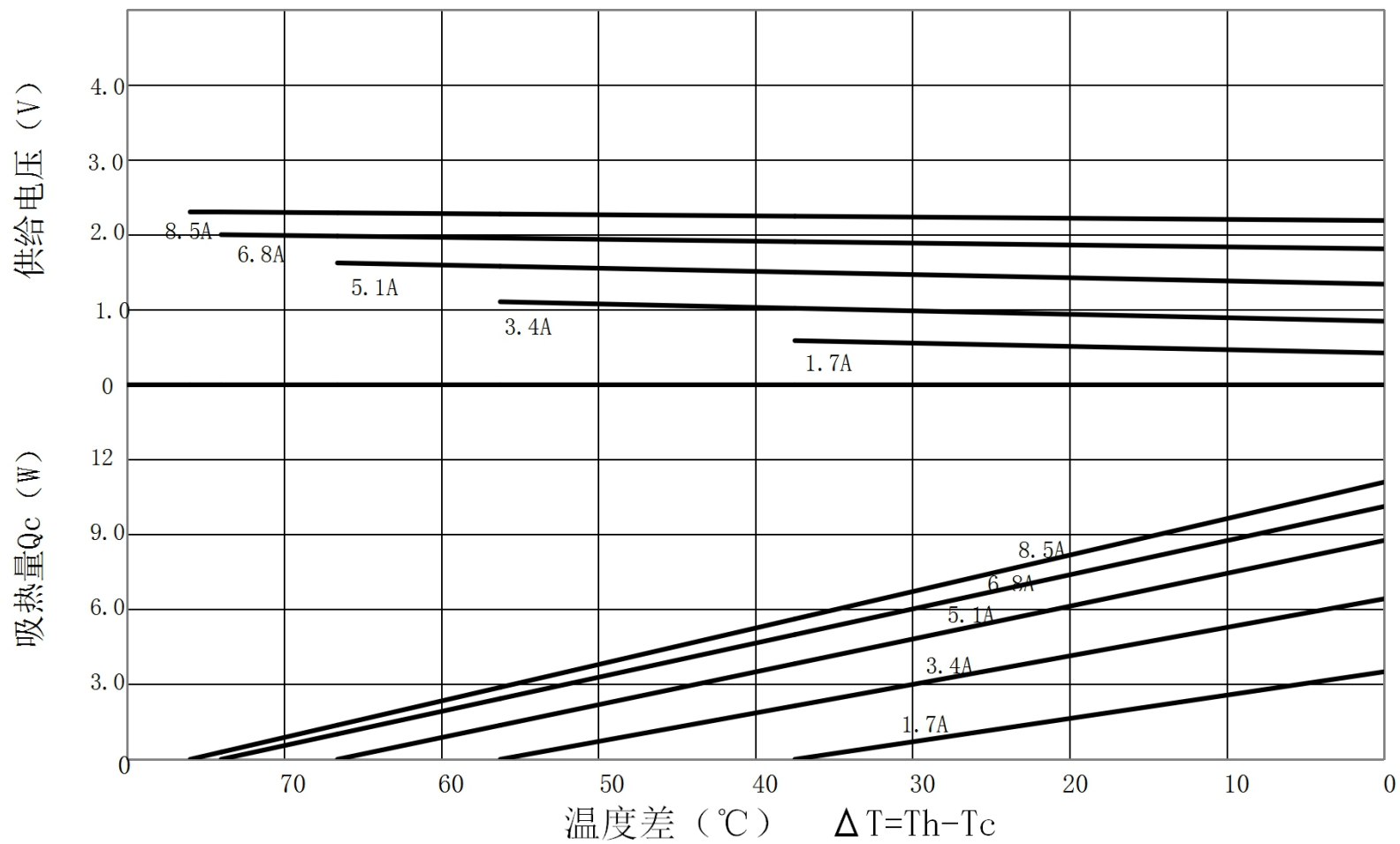
TEC1-B1708NC 特性图 (Th=50°C)
