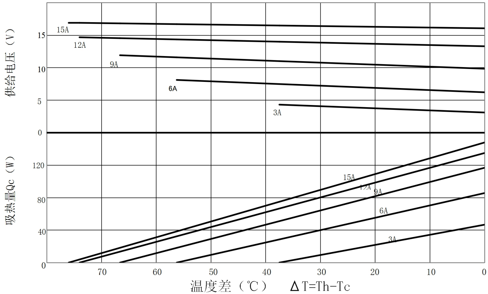
TEC1-B12715AC 特性图 (Th=50°C)
