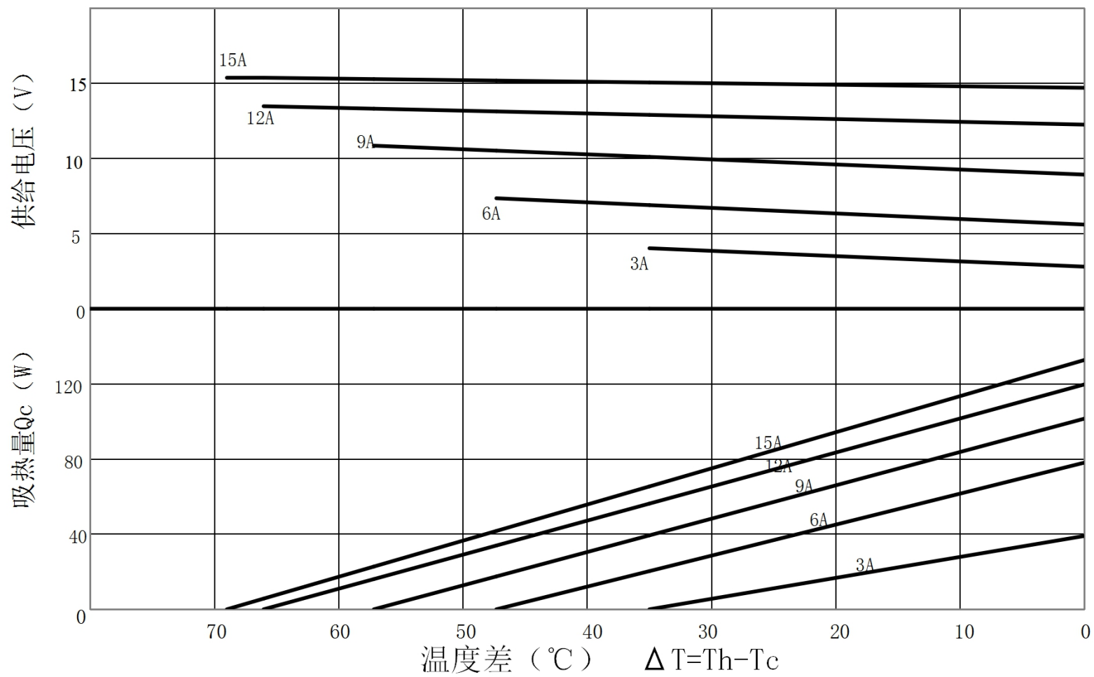
TEC1-B12715AC 特性图 (Th=27°C)
