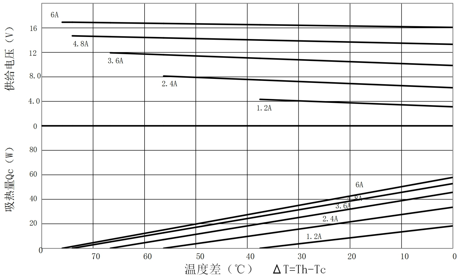
TEC1-B12706AC特性图 (Th=50°C)
